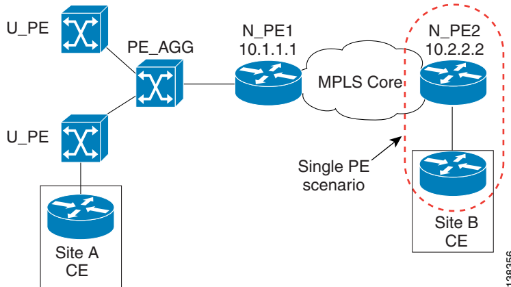
Figure D-2 Single PE scenario
