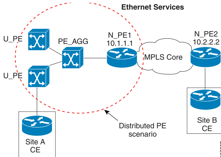
Figure D-3 Distributed PE Scenario
