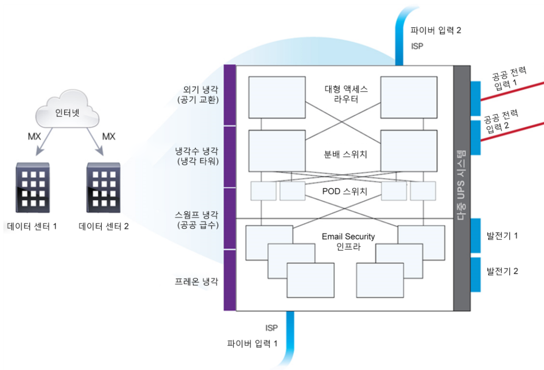
그림 2. Cisco Hosted Email Security 솔루션의 데이터 센터 아키텍처
