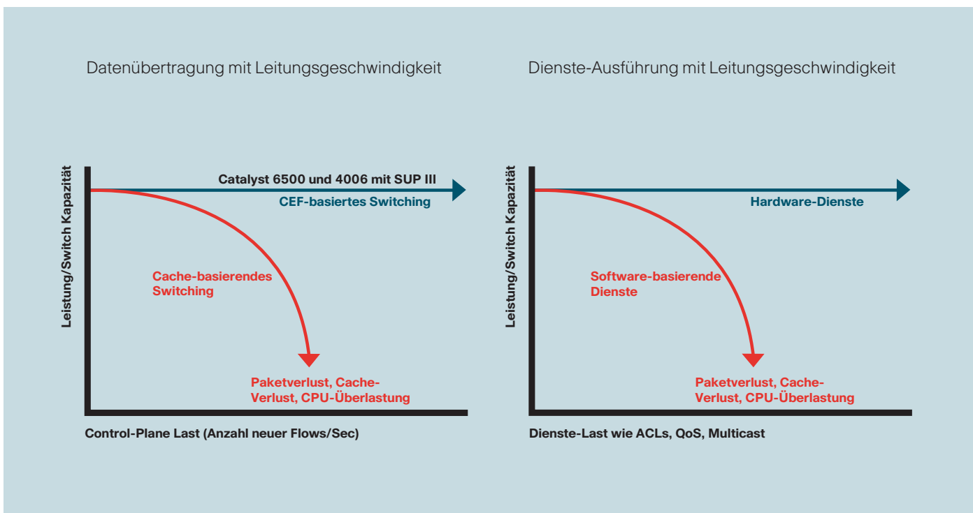
Abb. 3: Die Vorteile von Cisco Express Forwarding
