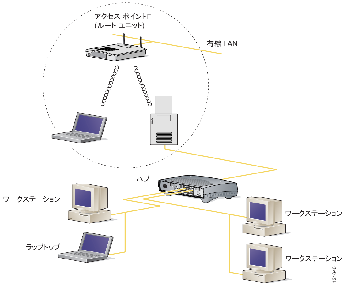
図 18-2 ワークグループ ブリッジ モードのアクセス ポイント
