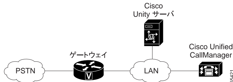
図 30-1 電話機システムと Cisco Unity の接続
