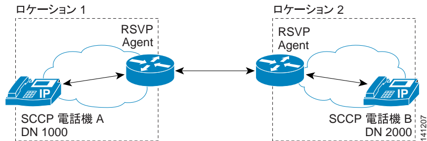
図 7-8 RSVP Agent 接続による電話機 A から電話機 B へのコール
