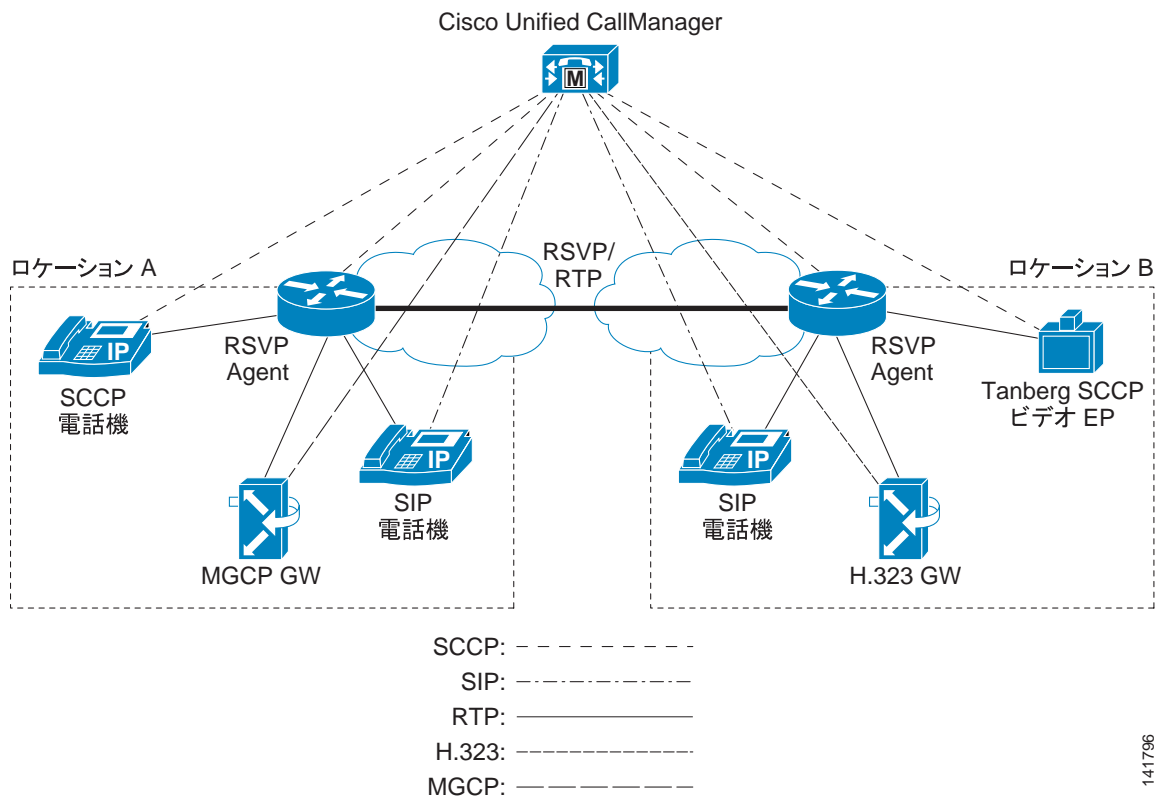
図 7-1 RSVP Agent を使用して設定された Cisco Unified Communications Manager ネットワーク
