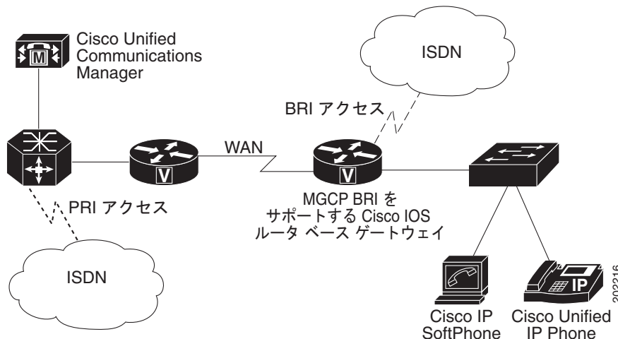
図 32-1 MGCP BRI インターフェイスを使用するトポロジのシナリオ
