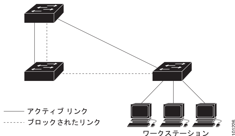
図 16-3 スパニング ツリーおよび冗長接続
