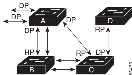
図 16-2 スパニング ツリー トポロジ
