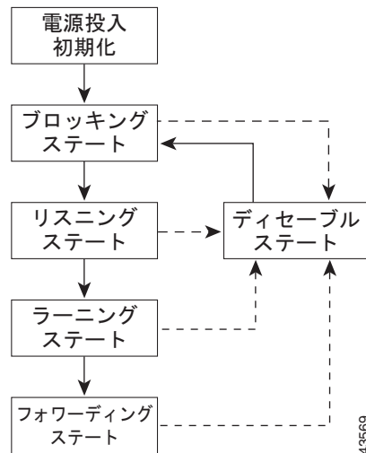
図 16-1 スパンニング ツリー インターフェイス ステート
