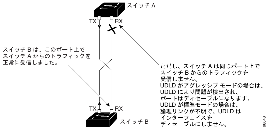
図 26-1 UDLD による単一方向リンク検出
