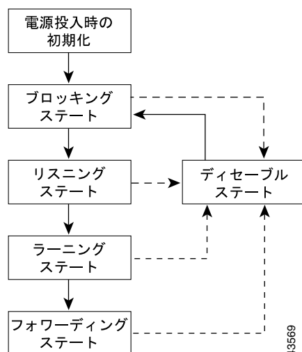
図 17-1 スパンニングツリー インターフェイスのステート
