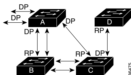
図 17-2 スパニングツリー トポロジ
