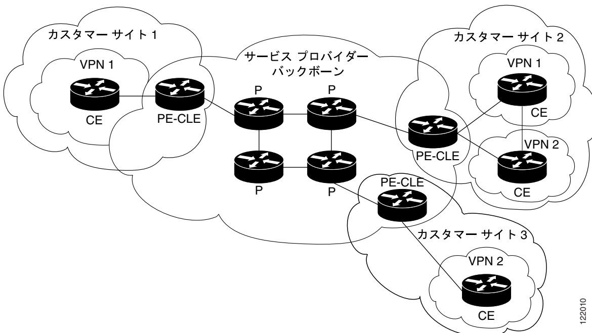
図 37-1 VPN およびサービス プロバイダー バックボーン
