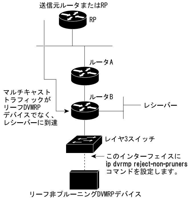
図 37-7 ルータが非プルーフ DVMRP ネイバを拒否する例
