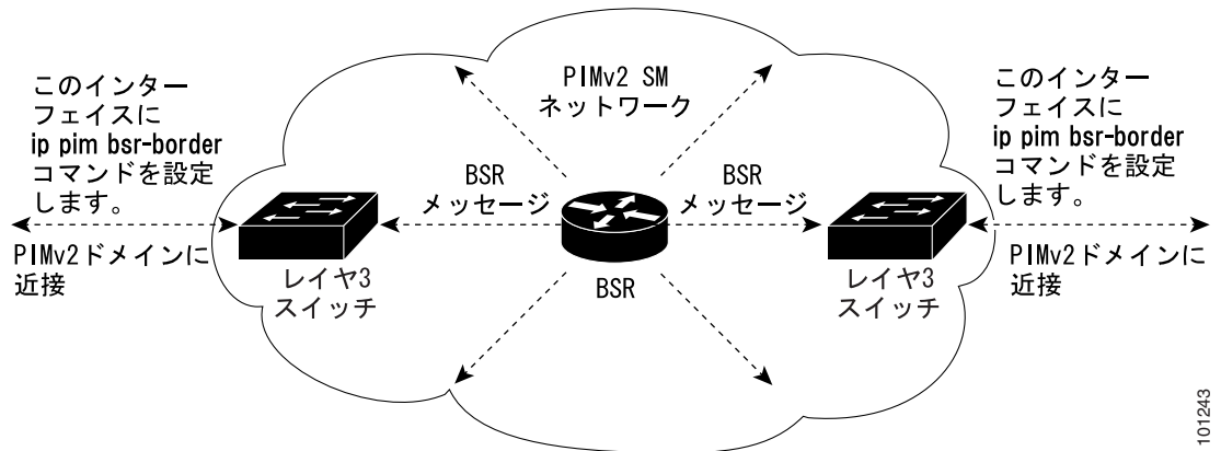
図 37-3 PIMv2 BSR メッセージの抑制
