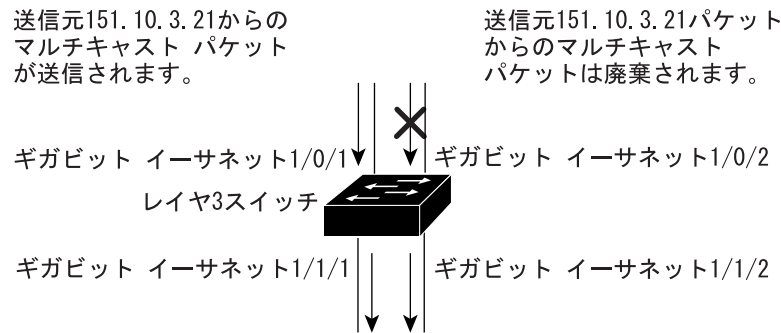
図 37-2 RPF チェック
