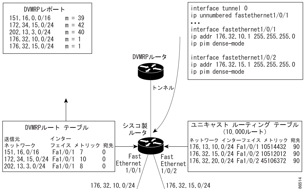
図 37-8 接続されたユニキャスト ルートにのみアドバタイズ (デフォルト) する例
