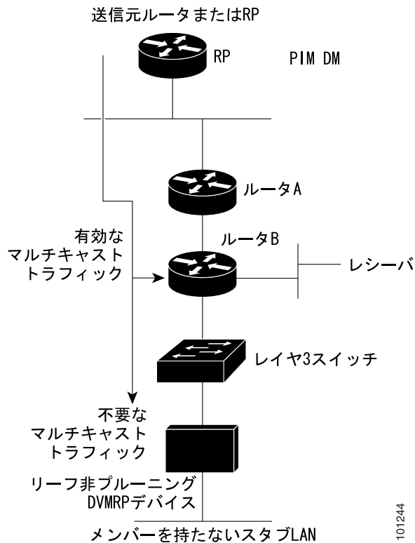
図 37-6 リーフの非プルーンング DVMRP ネイバ
