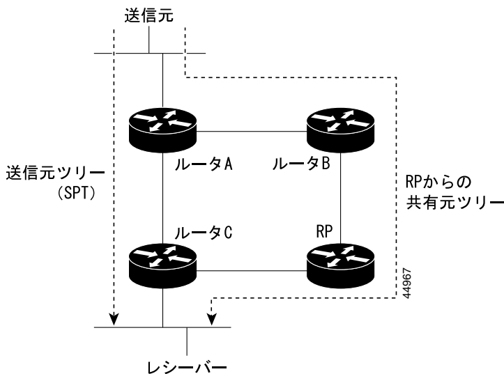
図 37-4 共有ツリーおよび送信元ツリー (SPT)
