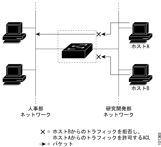
図 31-1 ACL によるネットワーク トラフィックの制御
