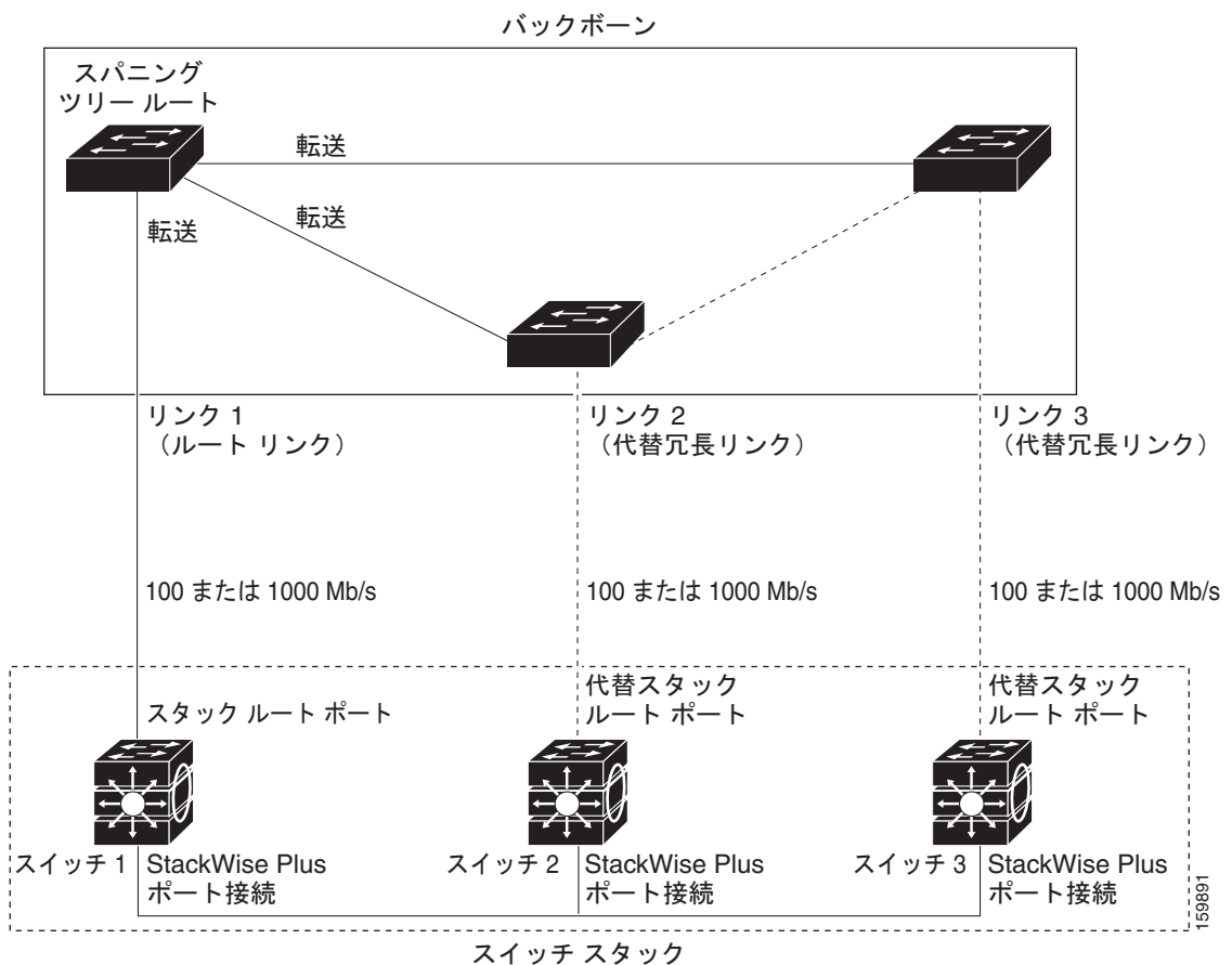
図 21-5 クロススタック UplinkFast トポロジ
