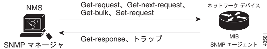
図 35-1 SNMP ネットワーク
