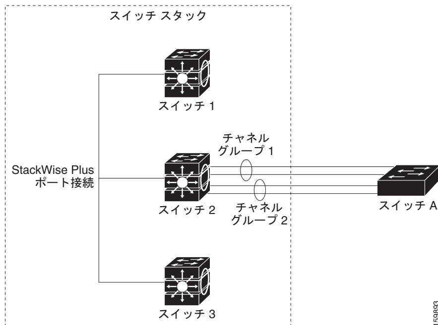
図 40-2 単一スイッチ EtherChannel
