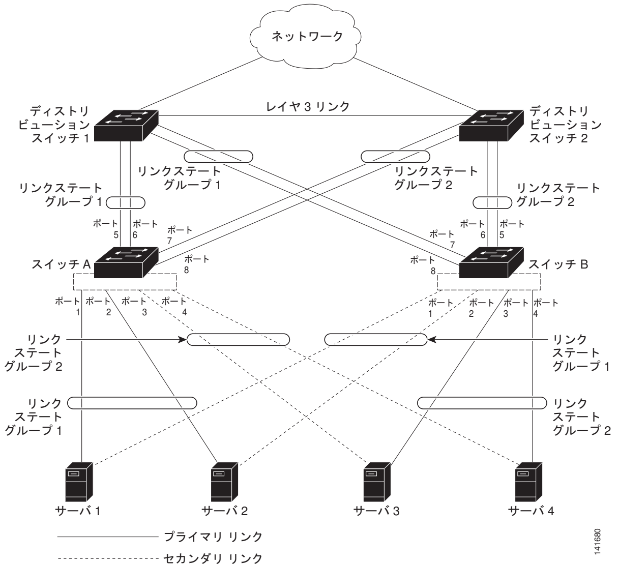
図 40-6 一般的なリンクステートトラッキングの設定
