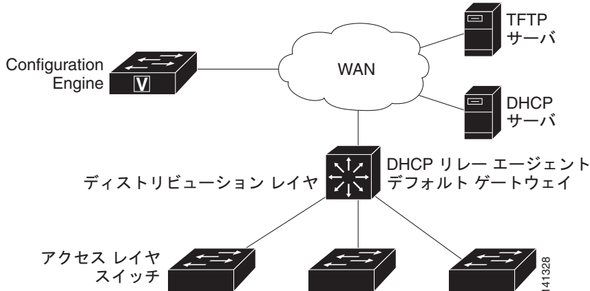
図 3-2 初期設定の概要
