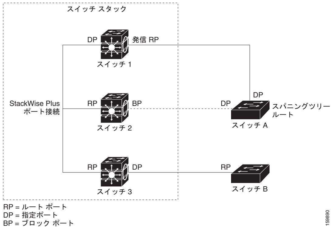
図 18-1 スイッチ スタックでのスパニング ツリー ポート ステート
