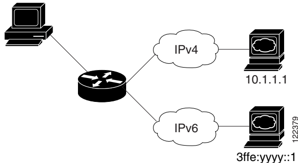
図 41-1 インターフェイス上での IPv4/IPv6 のデュアル サポート
