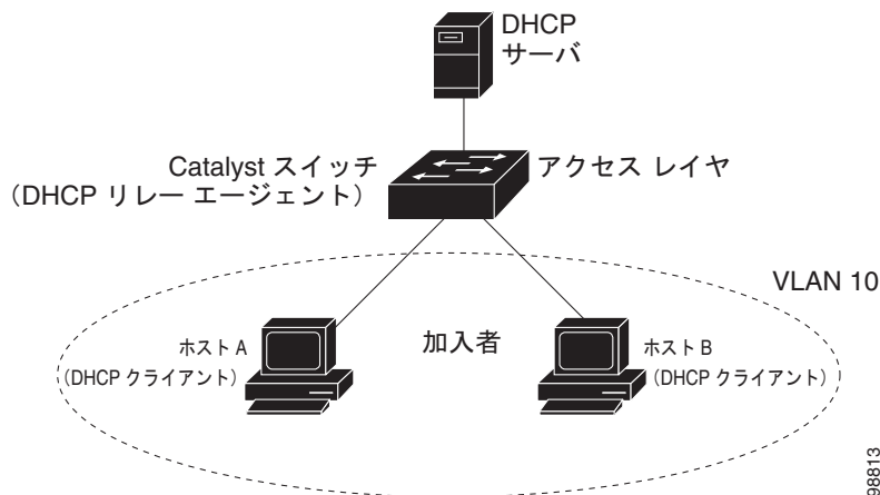
図 22-1 メトロポリタンイーサネット ネットワークにおける DHCP リレー エージェント
