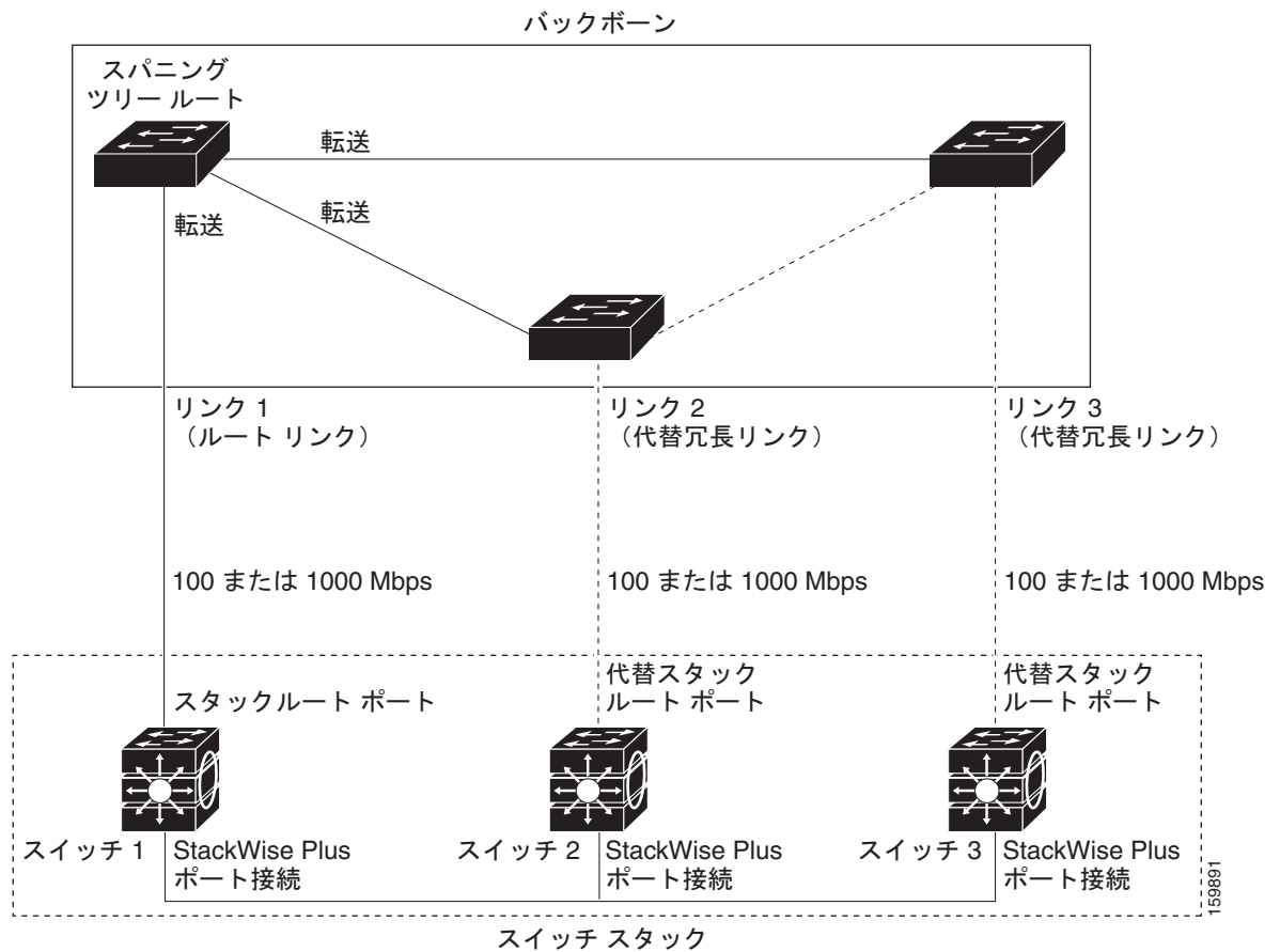
図 20-5 CSUF のトポロジ
