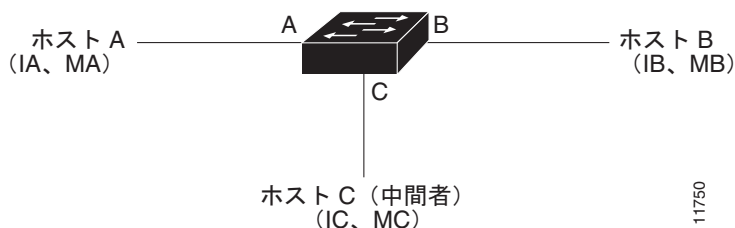
図 22-1 ARP キャッシュ ポイズニング
