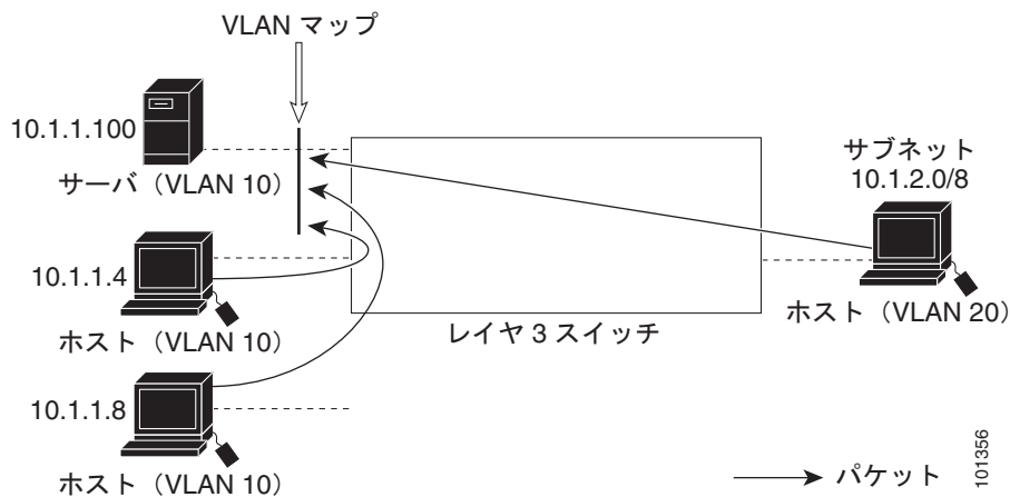
図 35-4 別の VLAN にあるサーバへのアクセス拒否
