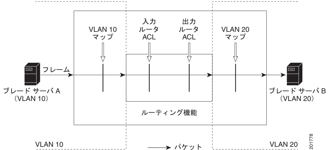
図 35-7 ルーテッド パケットへの ACL の適用
