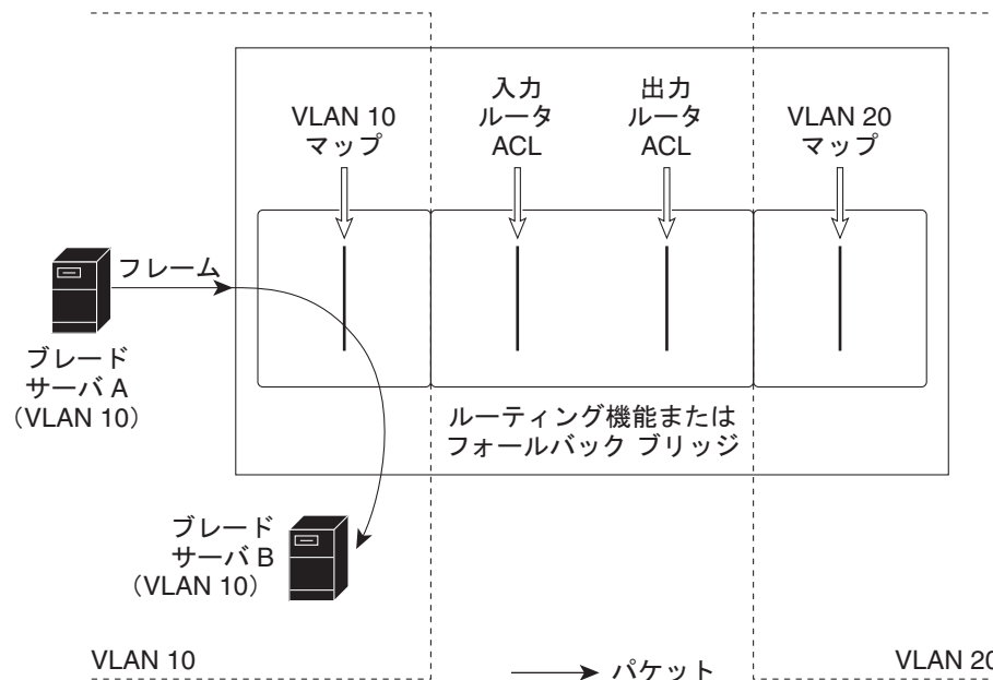
図 35-5 スイッチド パケットへの ACL の適用
