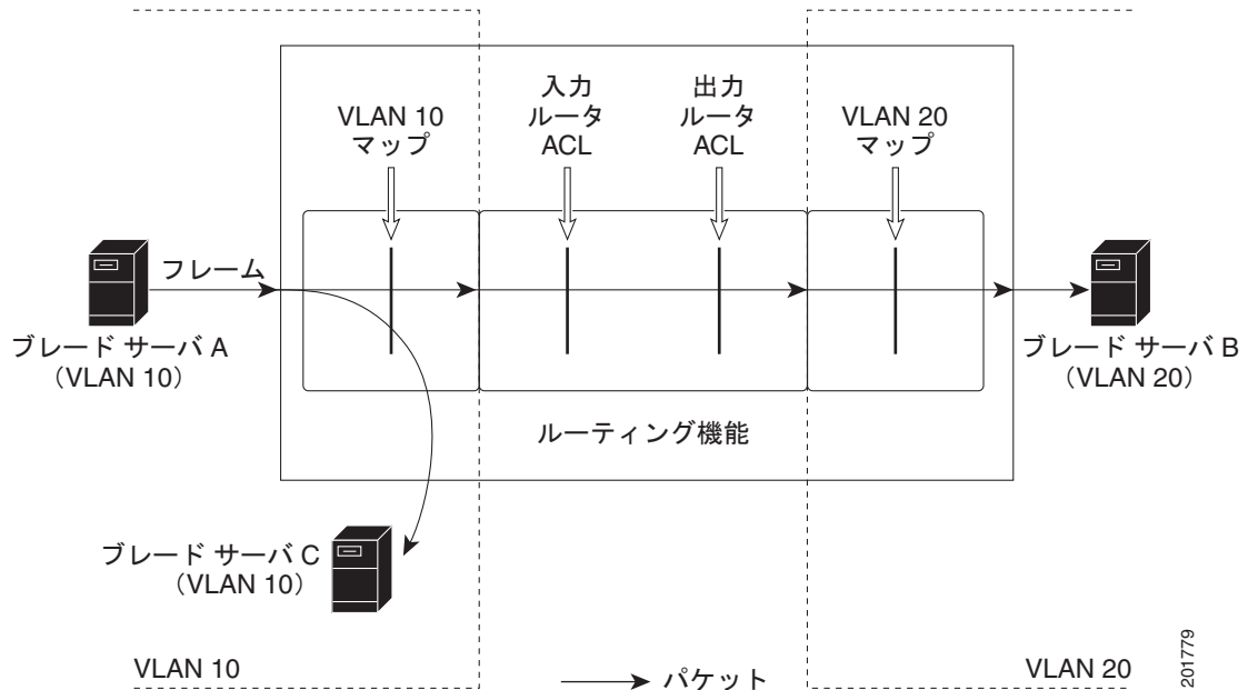
図 35-1 ACL を使用したネットワーク トラフィックの制御
