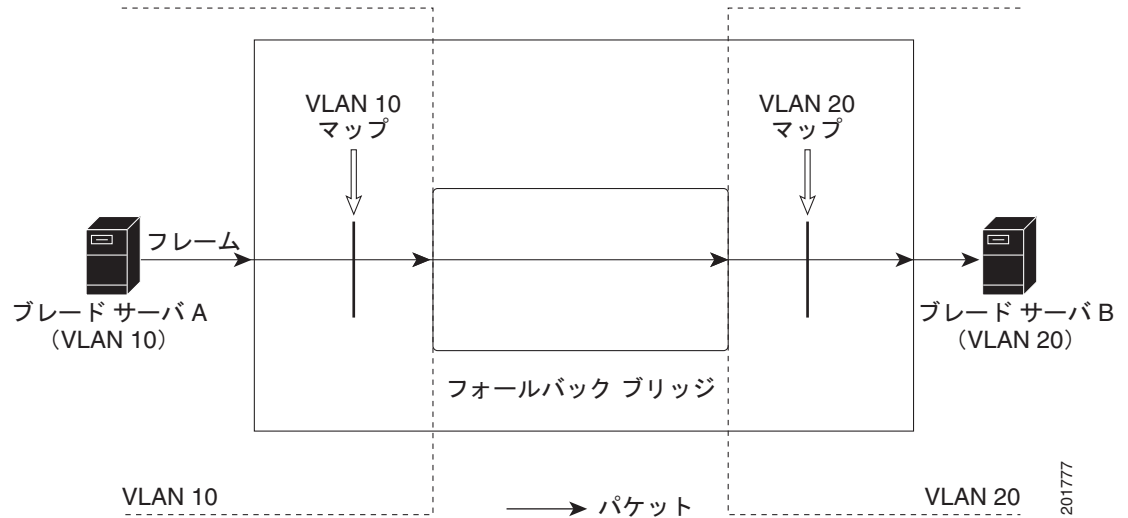
図 35-6 ブリッジド パケットへの ACL の適用
