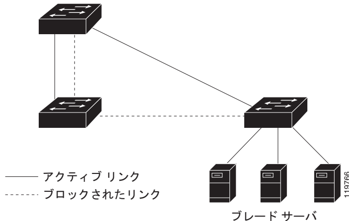
図 17-3 スパニング ツリーおよび冗長接続
