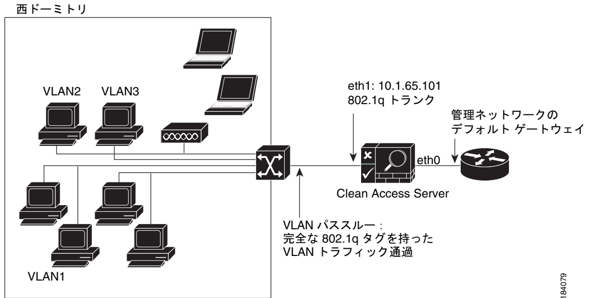
図 2-4 VLAN 対応ネットワーク内のブリッジング中央配置
