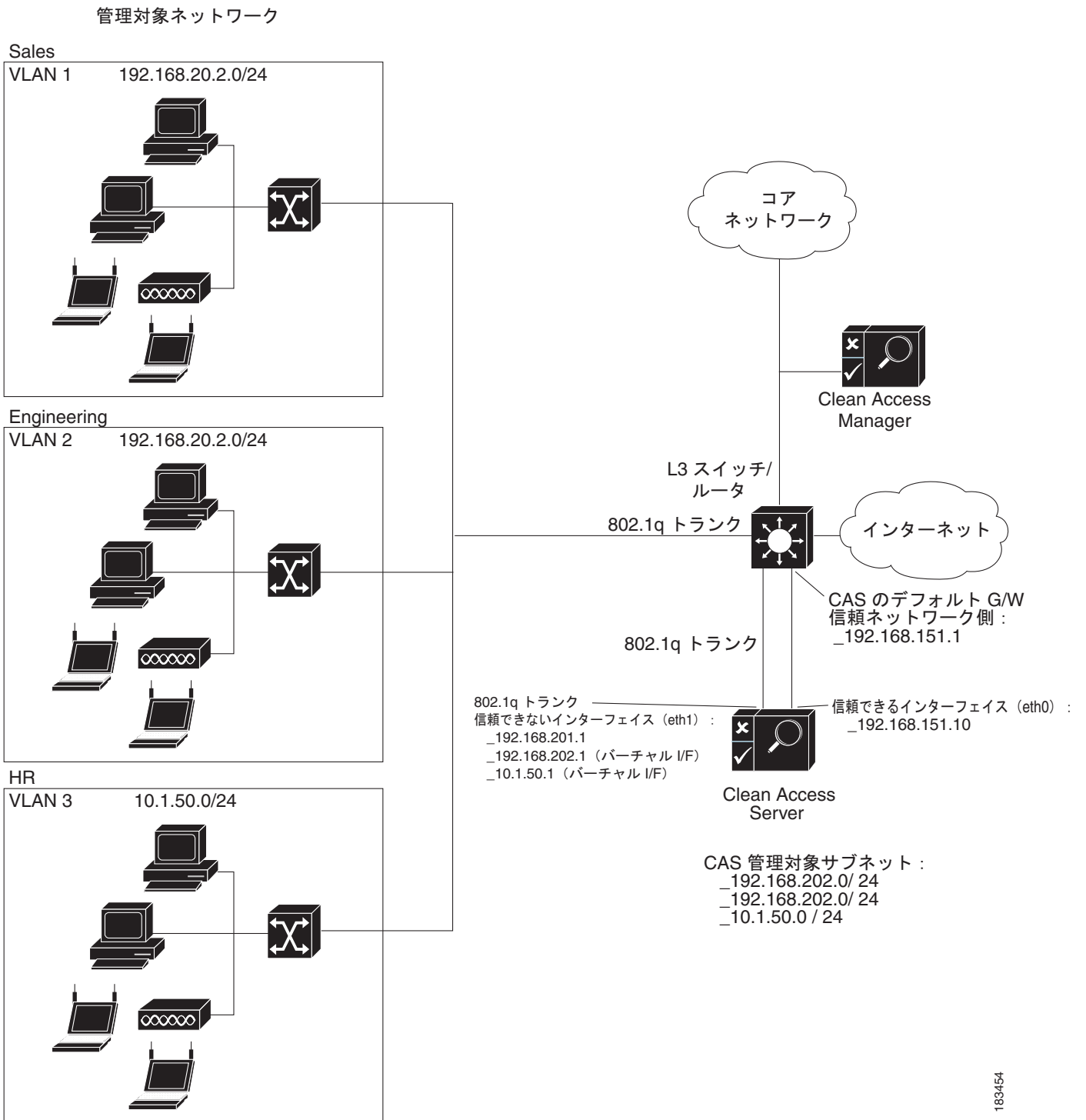
図 2-3 VLAN 対応ネットワークのルーテッド中央配置
