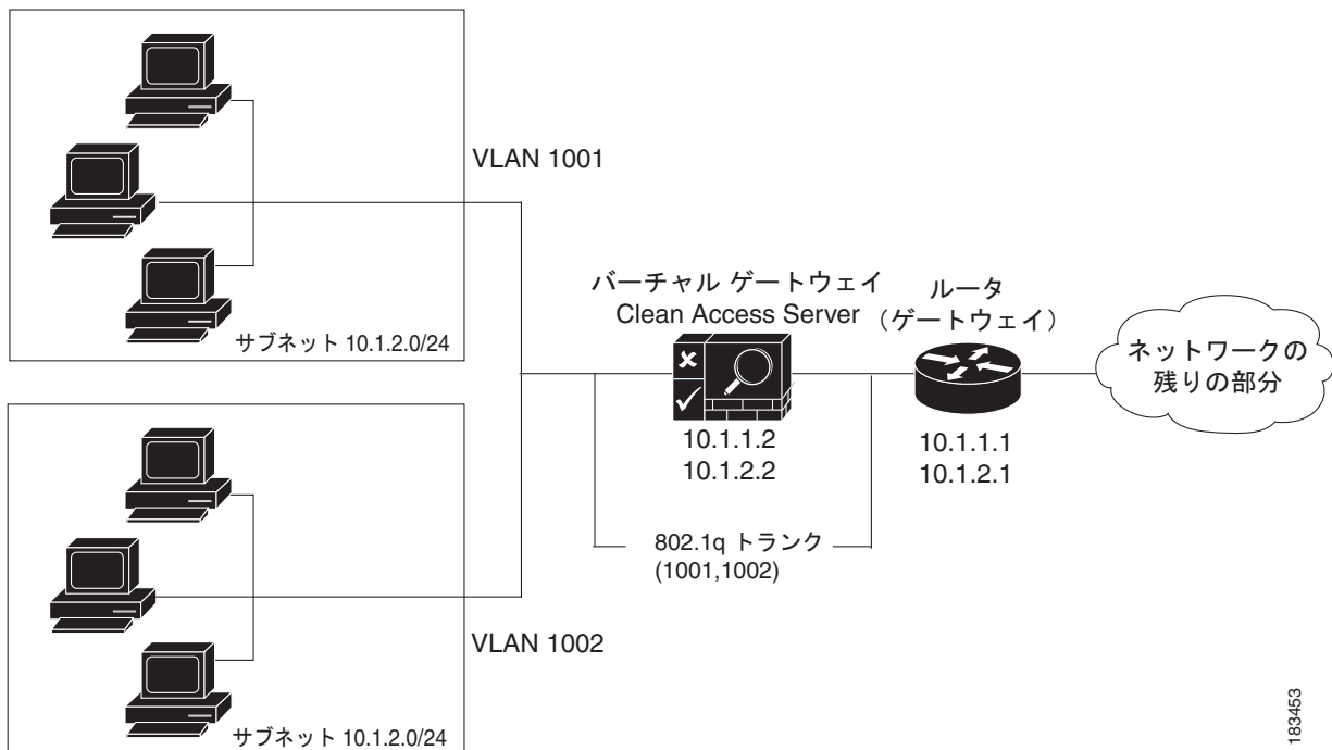
図 2-2 バーチャルゲートウェイの構成
