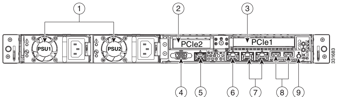
図 2-2 Cisco NAC ゲスト サーバの背面パネル (NAC-3415)
