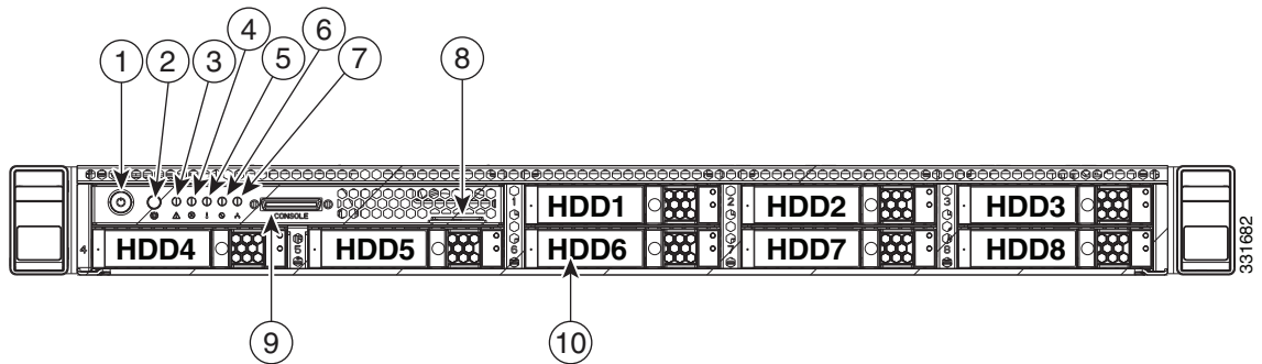
図 2-1 Cisco NAC ゲスト サーバの前面パネル (NAC-3415)
