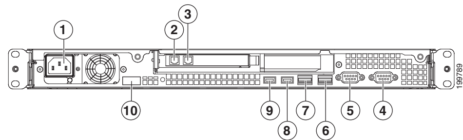
図 2-4 Cisco NAC ゲスト サーバの背面パネル (NAC-3315)
