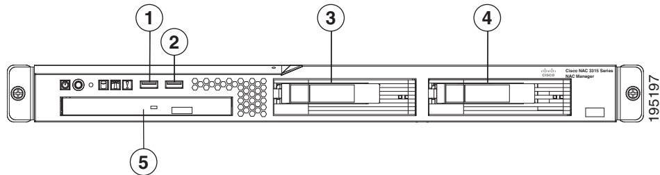
図 2-3 Cisco NAC ゲスト サーバの前面パネル (NAC-3315)
