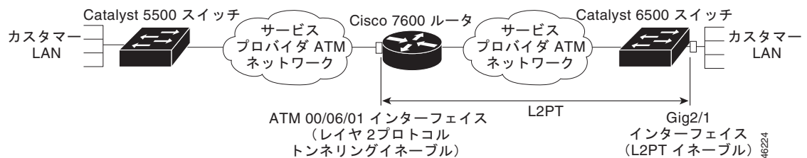
図 6-6 ATM SPA データのアーキテクチャ
