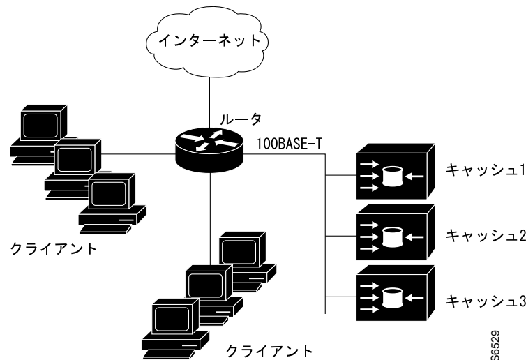
図 44-1 WCCP-Version 1 による Cisco Cache Engine ネットワークの設定
