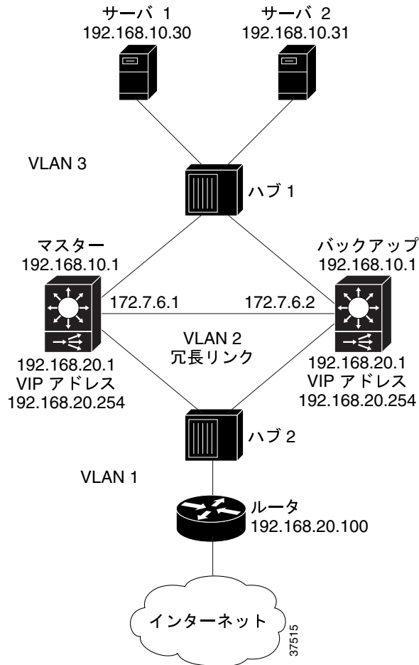
図 3-3 ステートレス冗長フェールオーバーのためのボックスツーボックス冗長性の例
