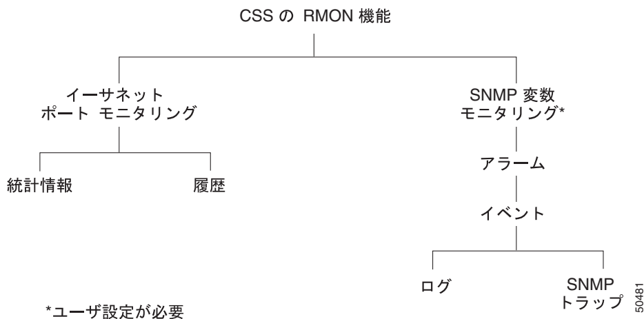
図 6-1 CSS でサポートされる RMON 機能
