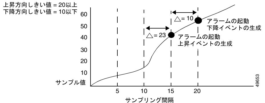
図 6-3 デルタ値サンプリングの例
