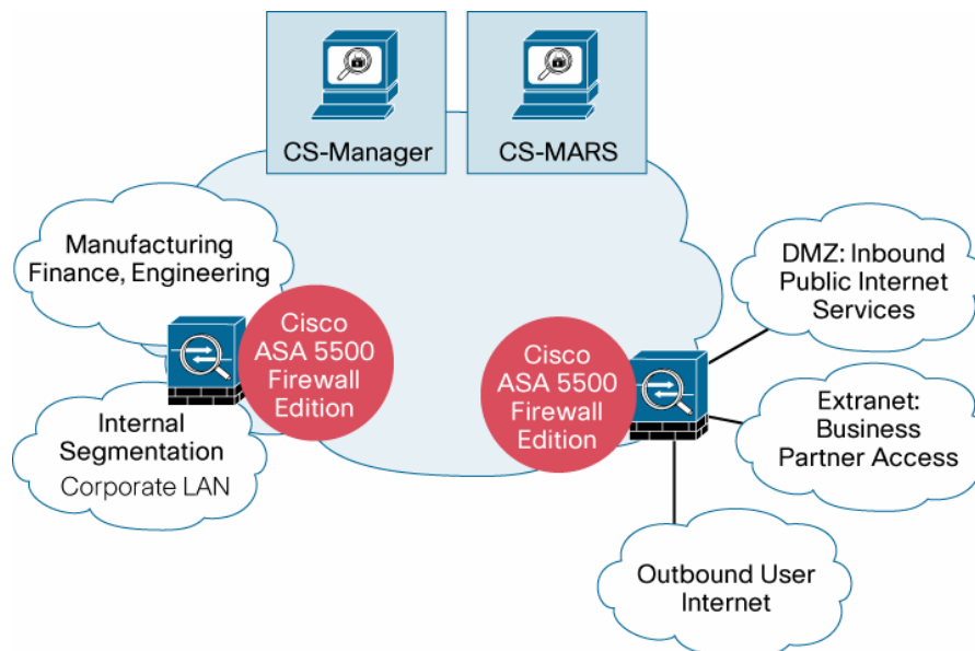
図1 ソリューション アーキテクチャ
