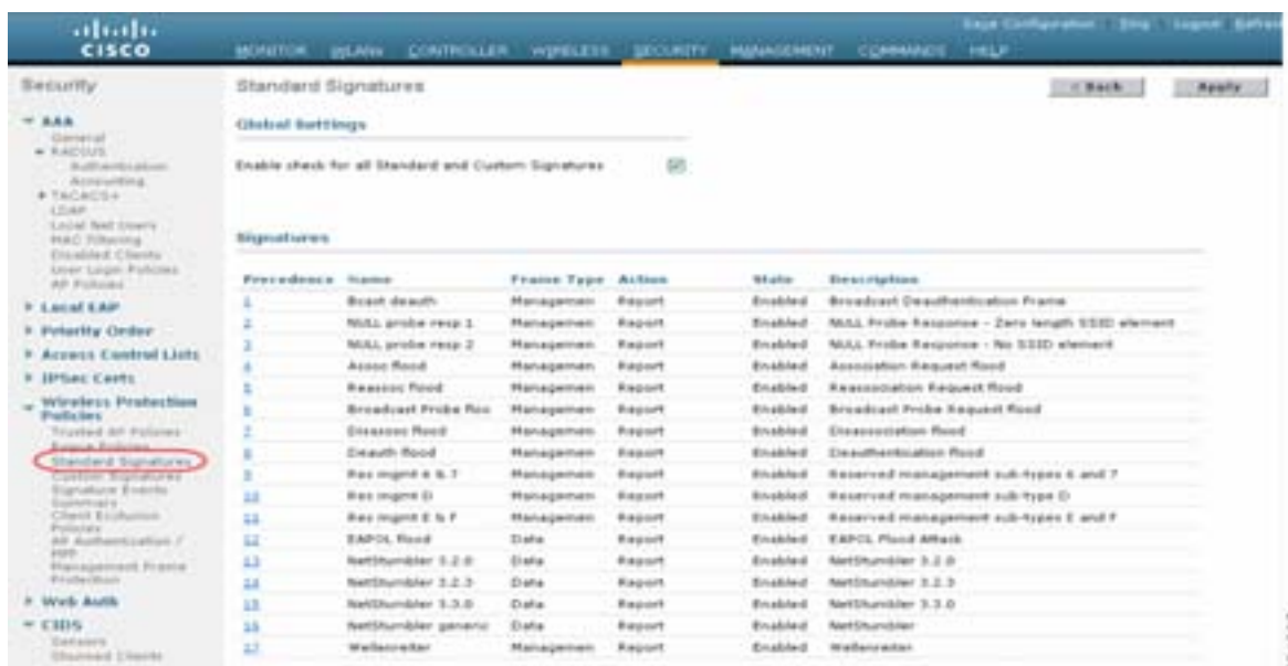
図 4-22 標準の WLAN IDS シグニチャ
