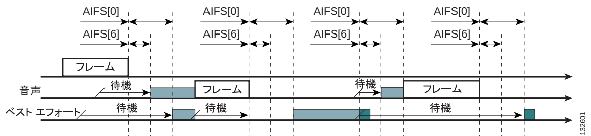
図 5-9 EDCA の例
