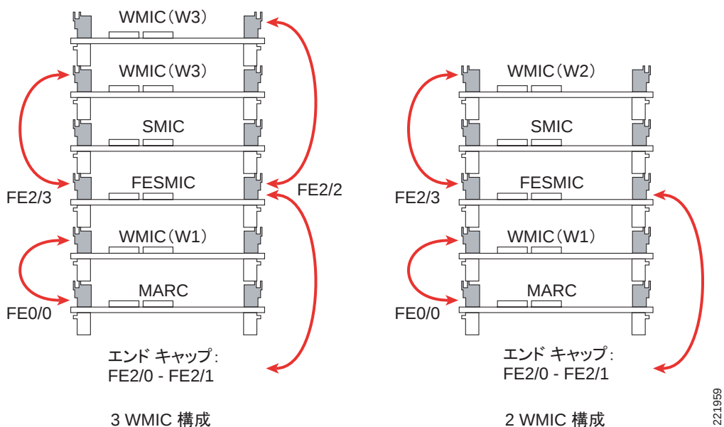
図 11-6 カードの接続
