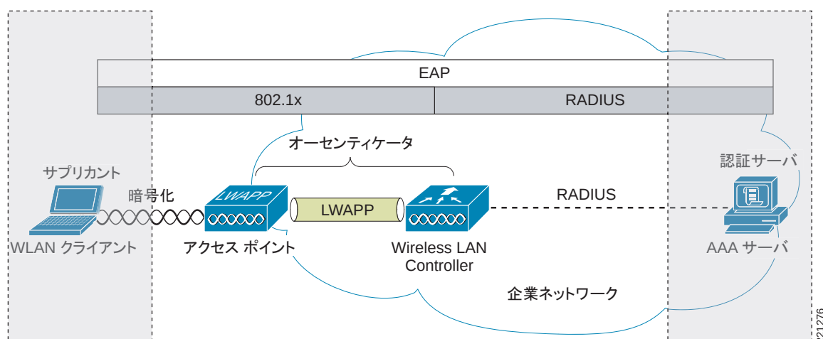
図 4-4 オーセンティケータの位置付け
