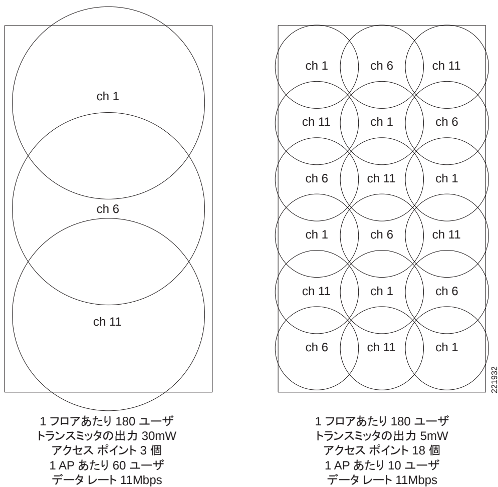
図 3-9 クライアント パフォーマンスを高めるために出力電力を変更
