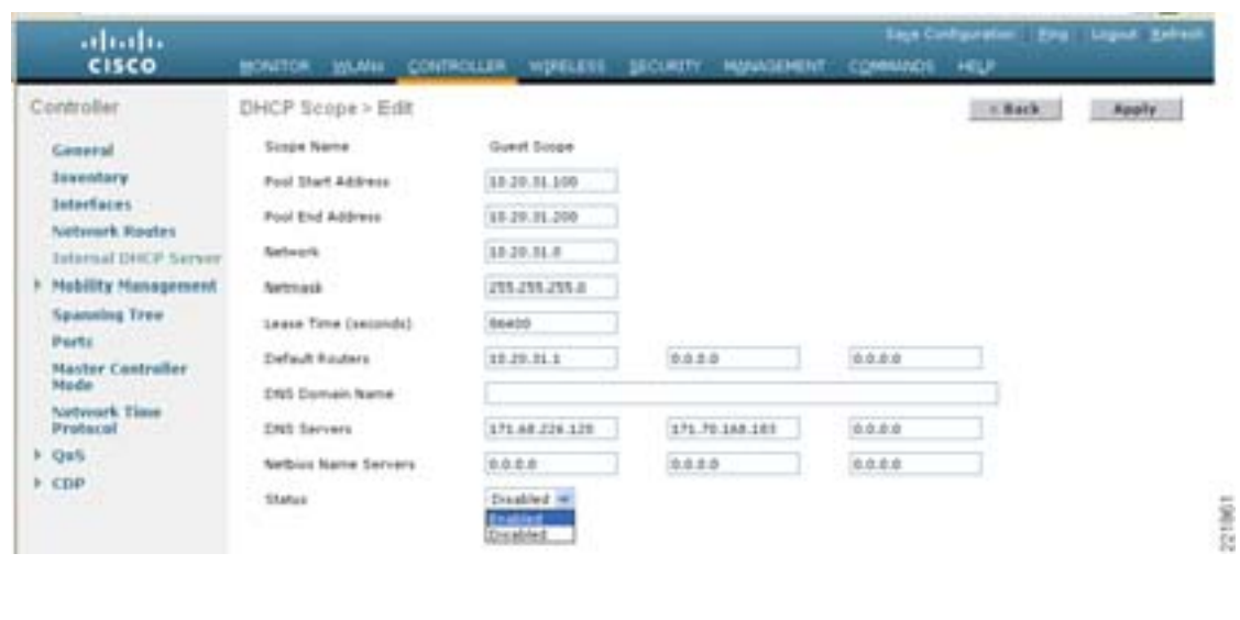
図 10-62 スコープ プロパティの設定と有効化
