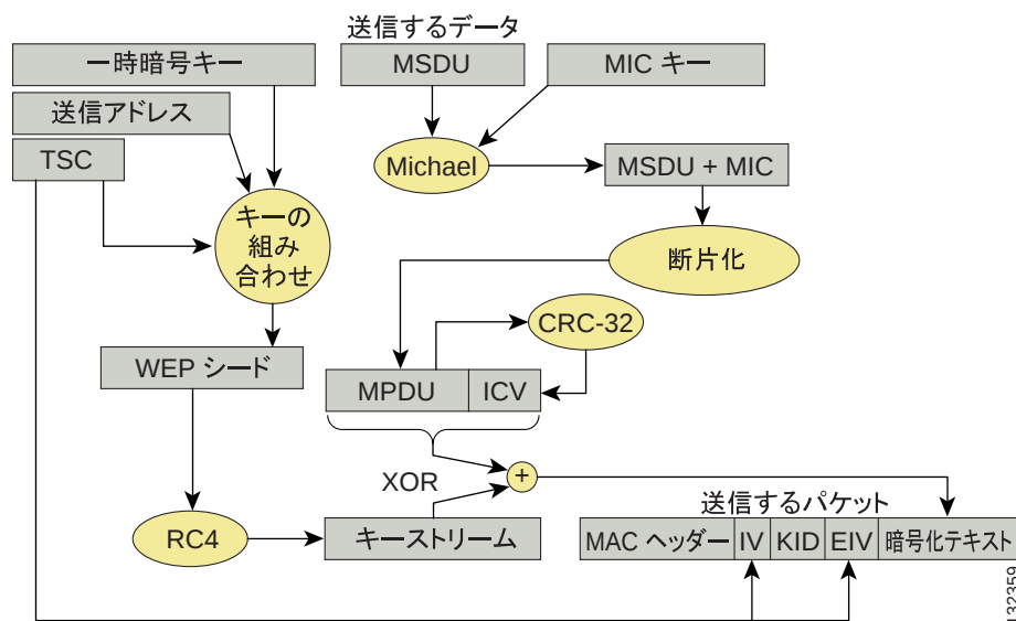
図 4-7 WPA TKIP
