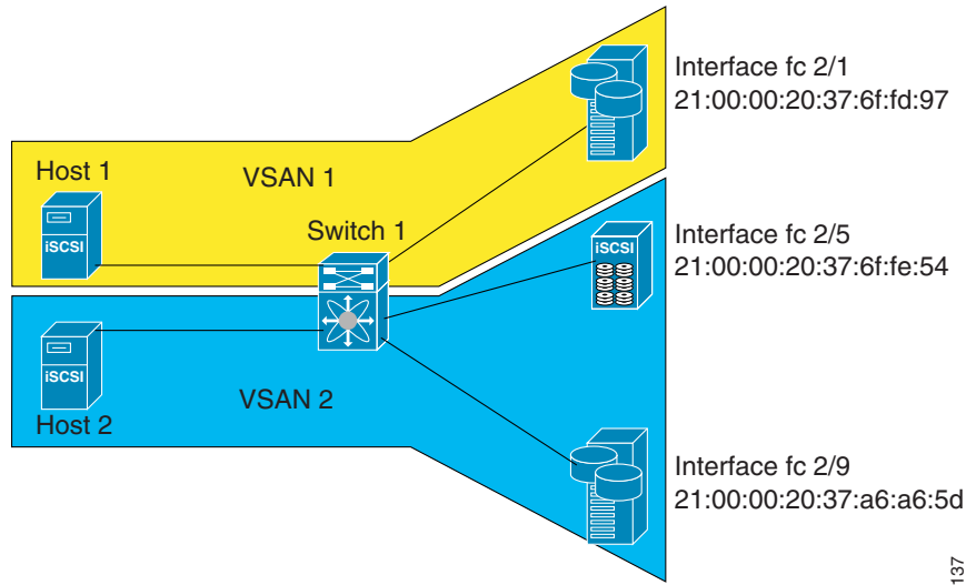
Figure 42-43 iSCSI Scenario 2
