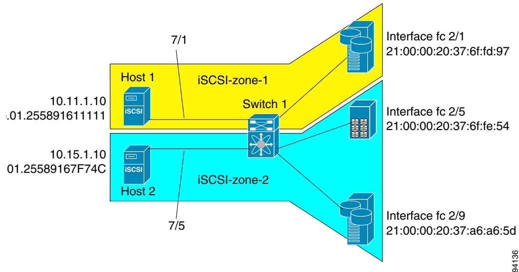
Figure 42-42 iSCSI Scenario 1
