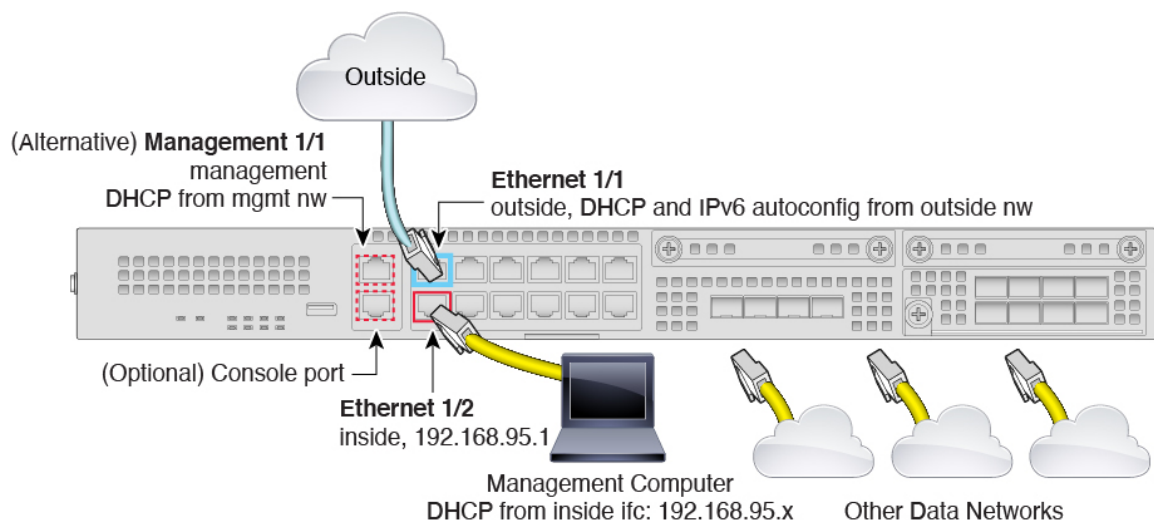
图 3: Firepower 2100 的布线
