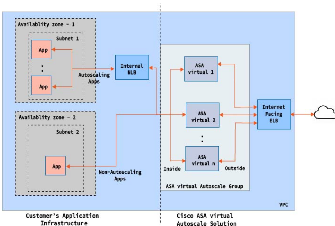
图 1: 使用三明治拓扑的 ASA 虚拟 Auto Scale 使用案例图
