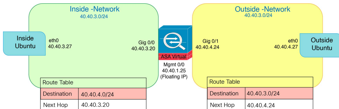
图 2: OpenStack 部署上的 ASA 虚拟 示例
