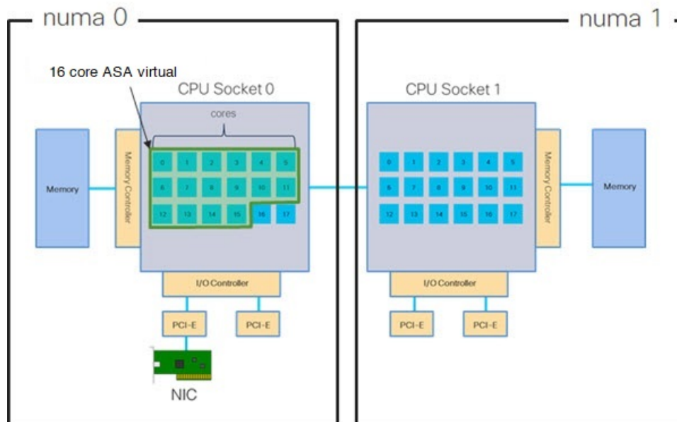
图 2: 16核 ASA 虚拟 NUMA 架构示例
