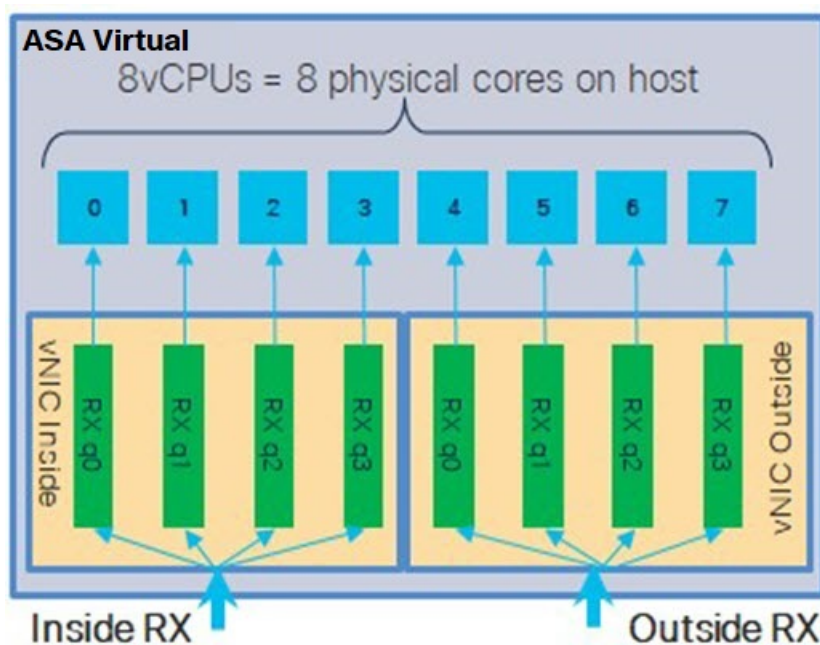
图 3: 8 核 ASA 虚拟 RSS RX 队列
