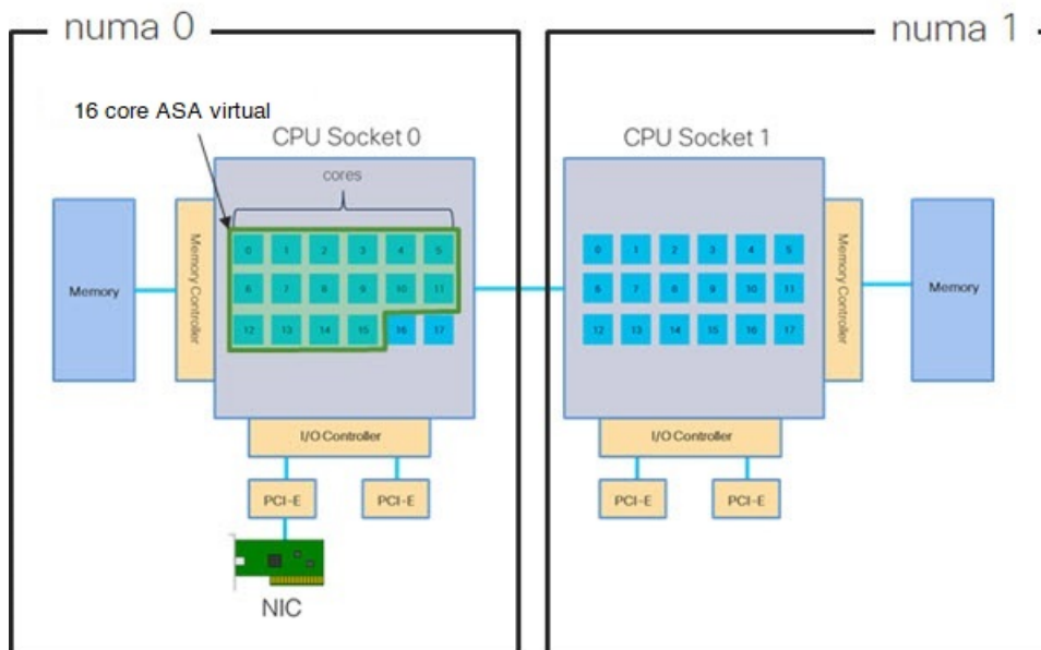
图 8: 16核 ASA 虚拟 NUMA 架构示例
