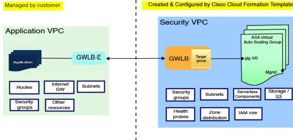
图 16: ASA 虚拟 AWS GWLB Auto Scale 使用案例图
