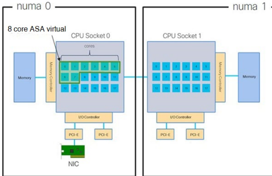
图 7: 8核 ASA 虚拟 NUMA 架构示例
