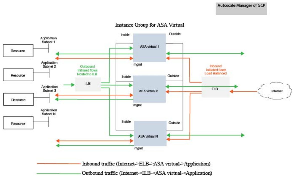
图 56: ASA 虚拟 Auto Scale 使用案例
