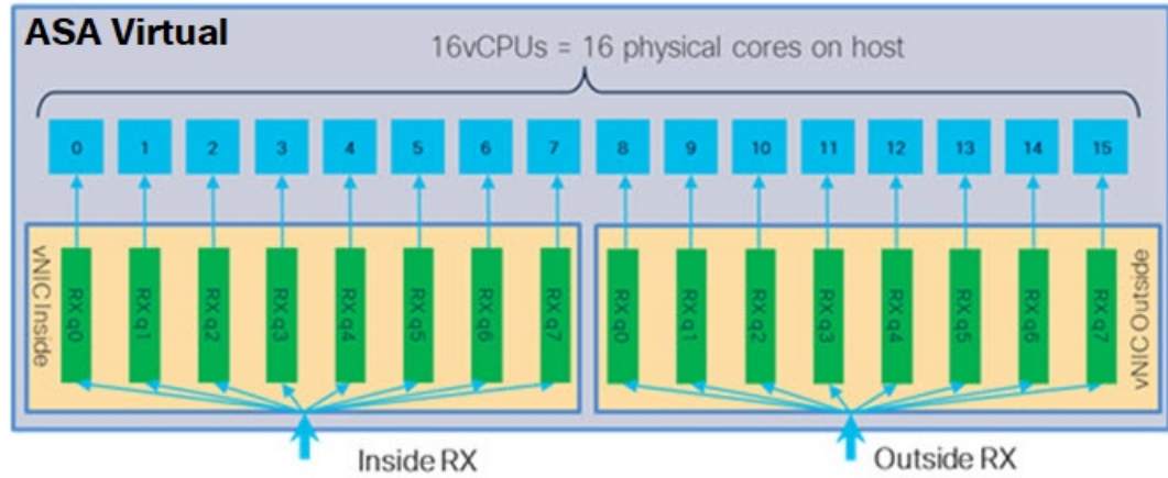
图 4: 16 核 ASA 虚拟 RSS RX 队列
