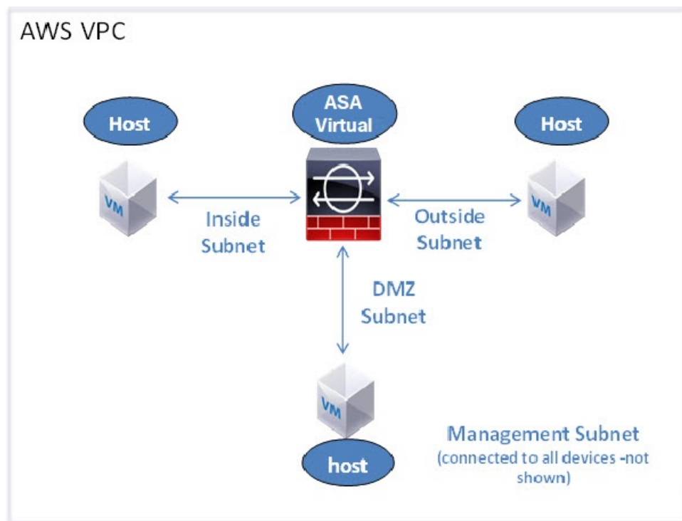
图 14: AWS 上的 ASA 虚拟部署示例
