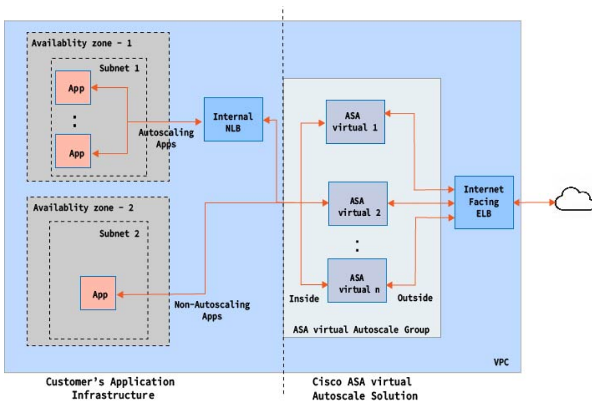
图 15: 使用三明治拓扑的 ASA 虚拟 Auto Scale 使用案例图
