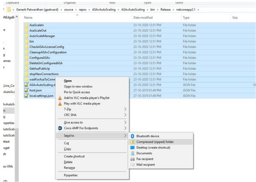
图 37: 生成 ASM_Function.zip
