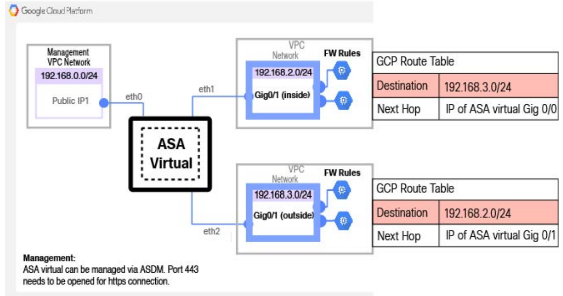
图 55: GCP 上的 ASA 虚拟部署示例
