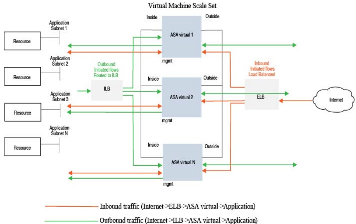
图 17: 使用三明治拓扑的 ASA 虚拟 Auto Scale 使用案例
