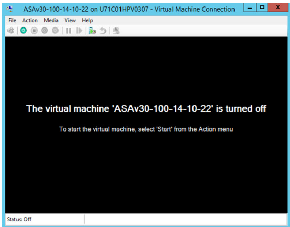
图 47: 启动虚拟机
