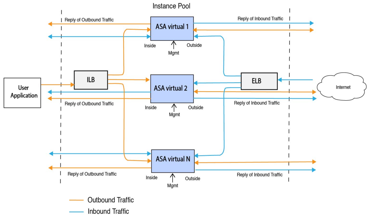
图 53: 使用案例图
