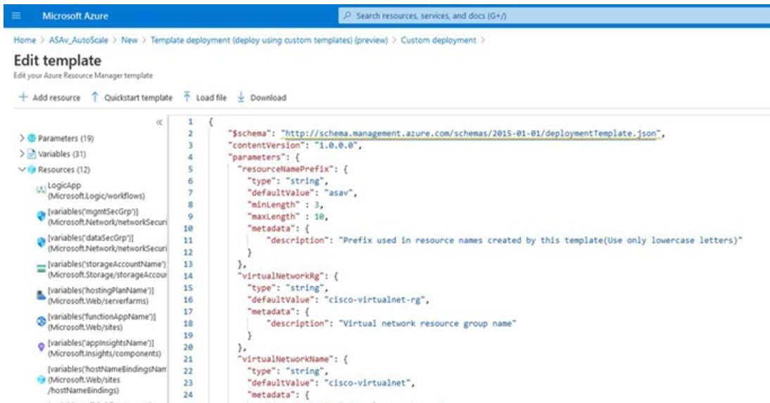
图 21: 编辑模板
