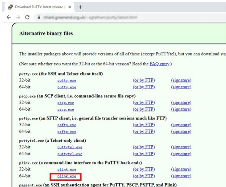
图 26: 下载 PuTTY
