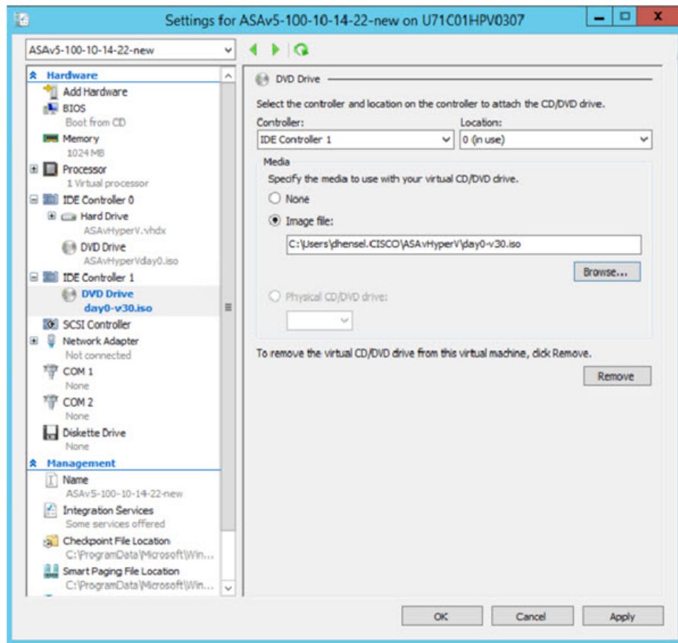
图 39: Hyper-V 管理器
