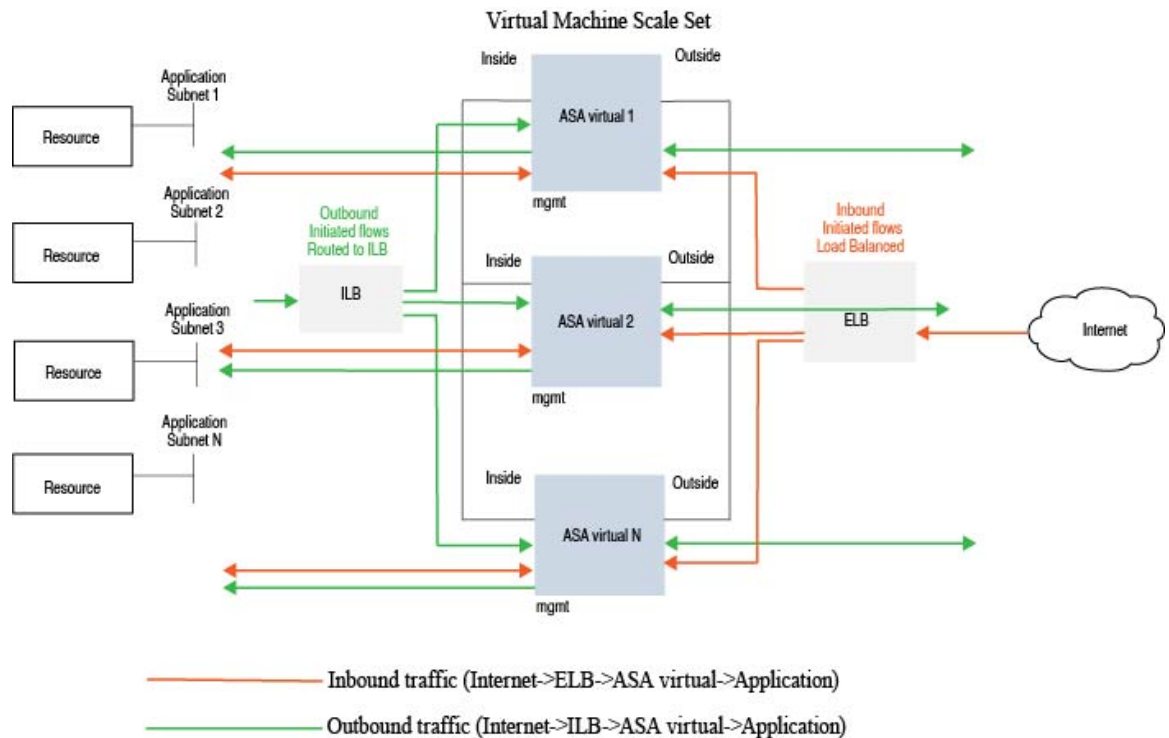
图 17: ASA 虚拟 Auto Scale 使用案例
