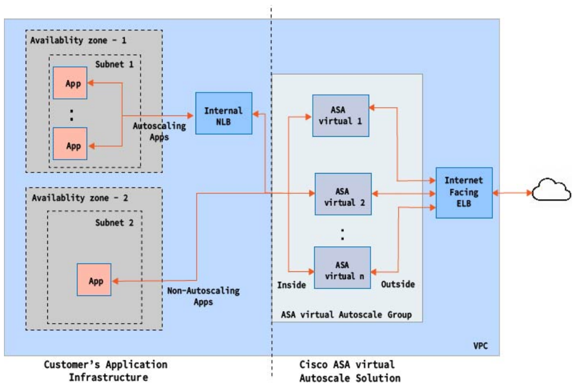
图 15: ASA 虚拟 Auto Scale 使用案例图
