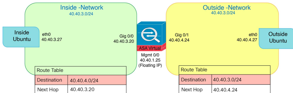
图 65: OpenStack 部署上的 ASA 虚拟示例
