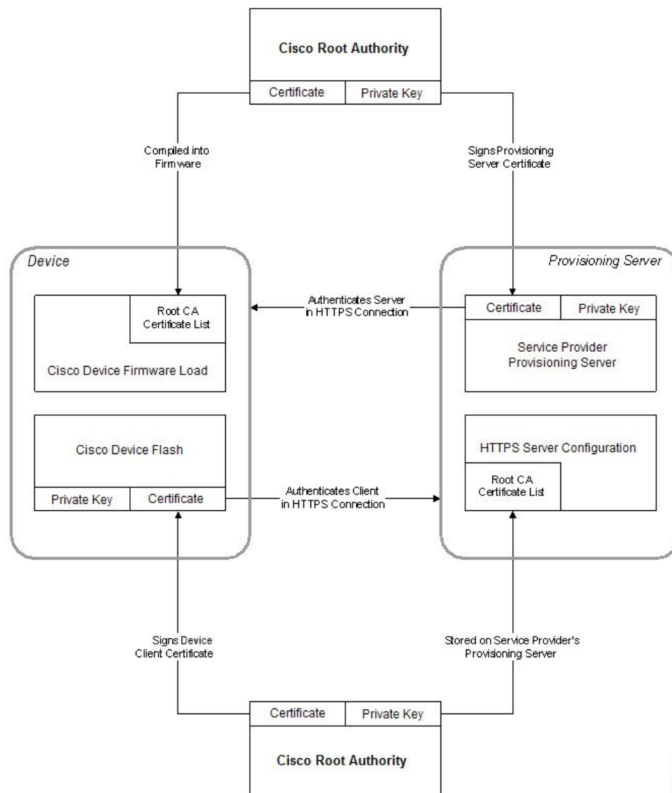
図 6: 認証局のフロー
