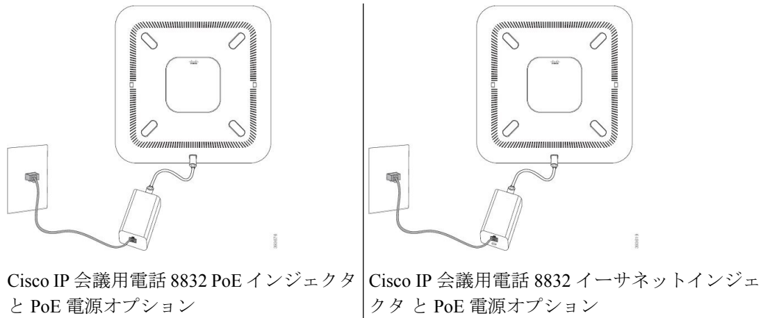
図 7: 会議用電話の PoE 電源オプション
