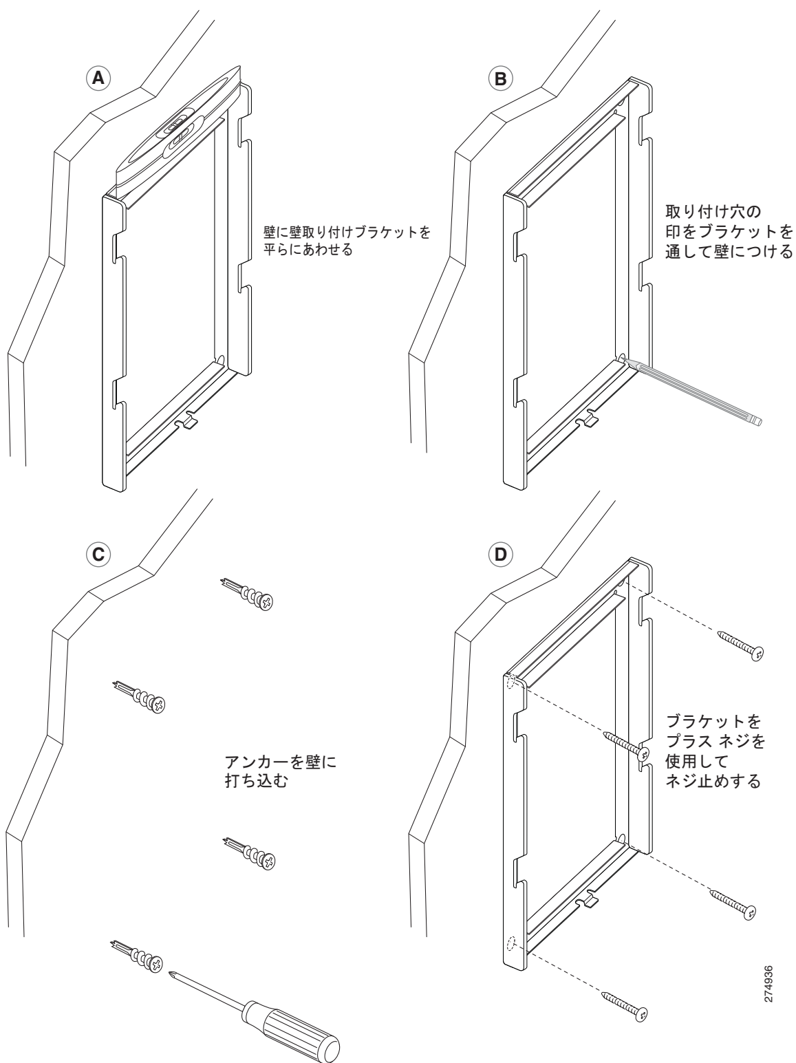
図 E-8 壁面用ブラケットの取り付け
