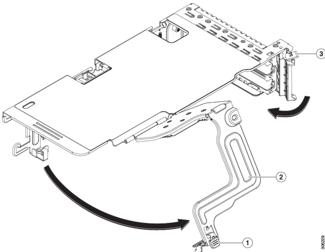
図 34: PCIe ライザーカードの固定機構
