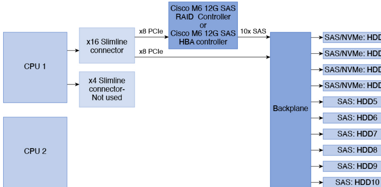
図 44: Cisco M6 12G SAS RAID または Cisco 12G SAS HBA コントローラを使用している Cisco UCS C225 M6 のブロック図
