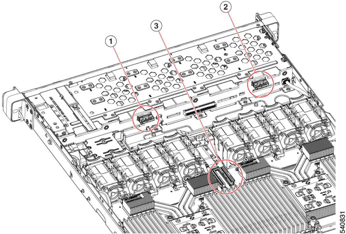
図 30: バックプレインの NVMe-B1 および B2、およびマザーボードの NVMe-B
