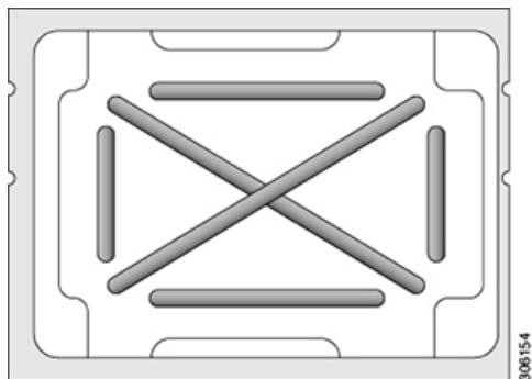
図 22: サーマル インターフェイス マテリアルの塗布パターン
