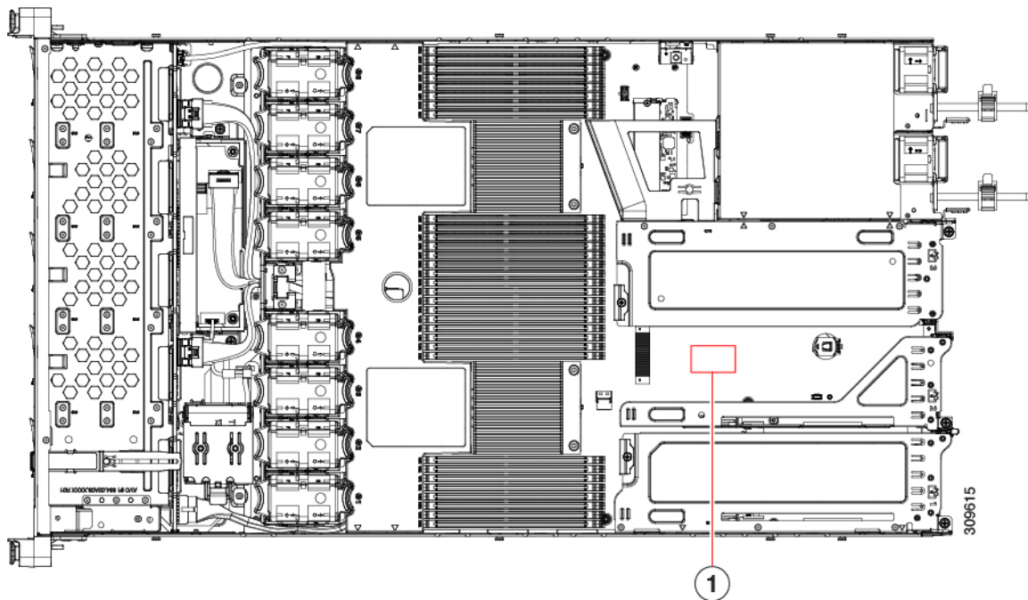
図 39: マザーボード上の TPM ソケットの位置
