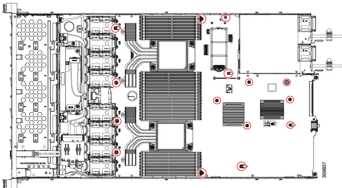
図 40: UCS C225 M6 PCBA を取り外すためのネジの位置
