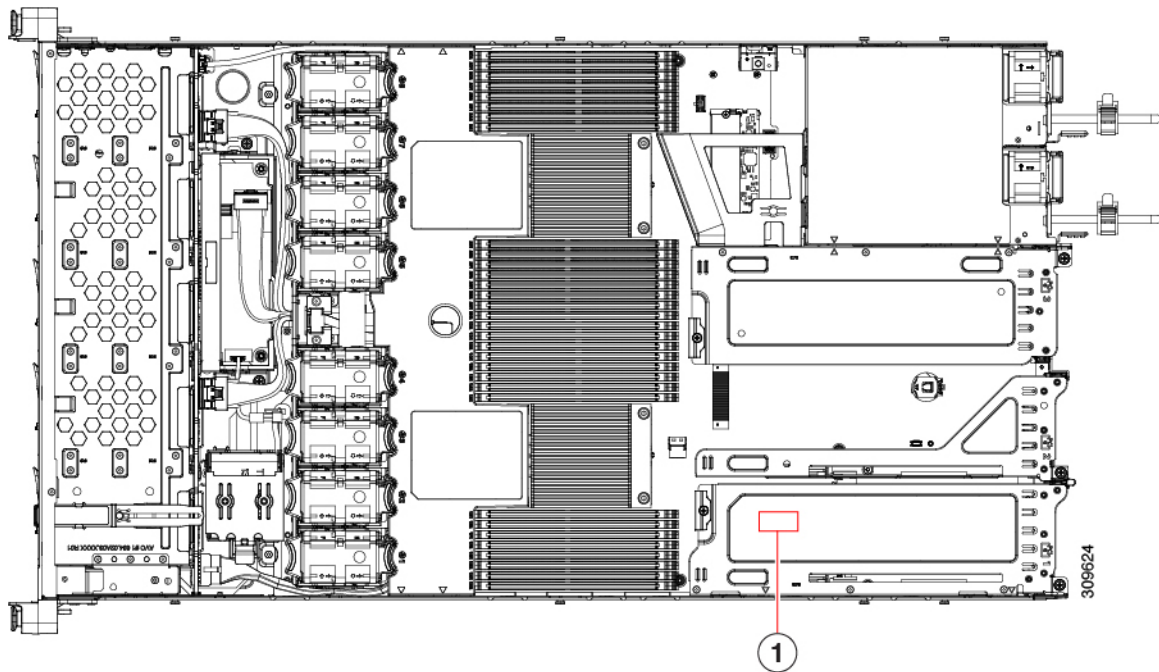
図 24: 内部 USB ポートの場所
