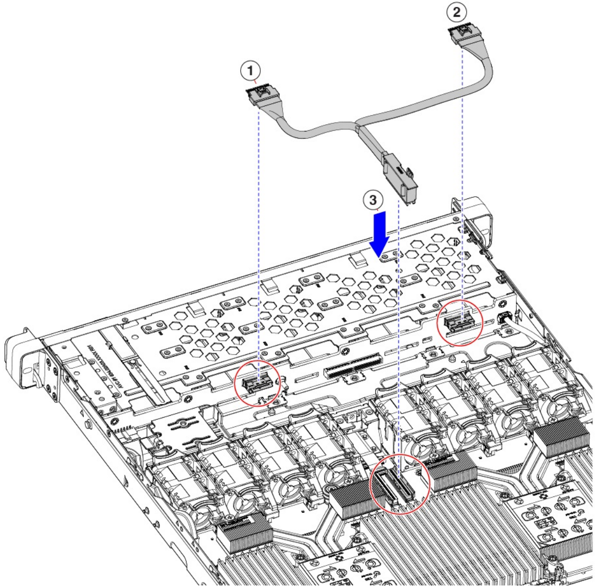
図 31: ケーブル コネクタ
