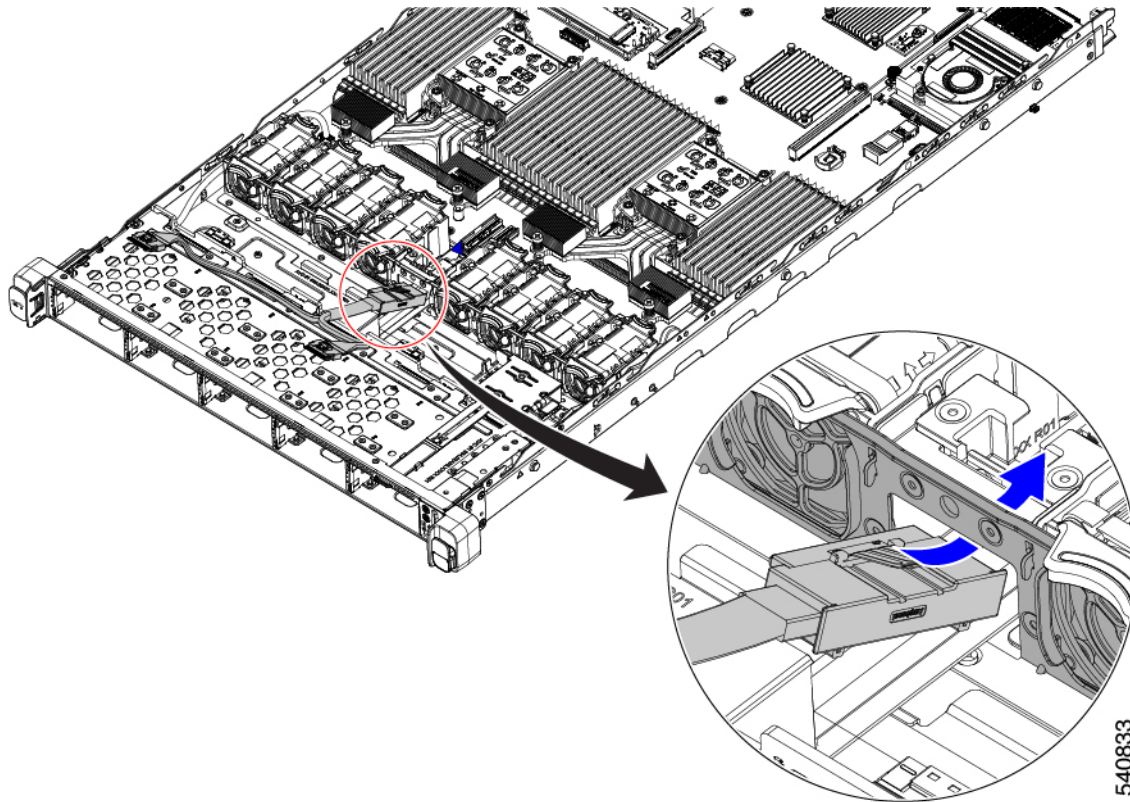
図 32: NVMe-B プラグをファン ケージの開いた穴に通し、マザーボードに挿入します。
