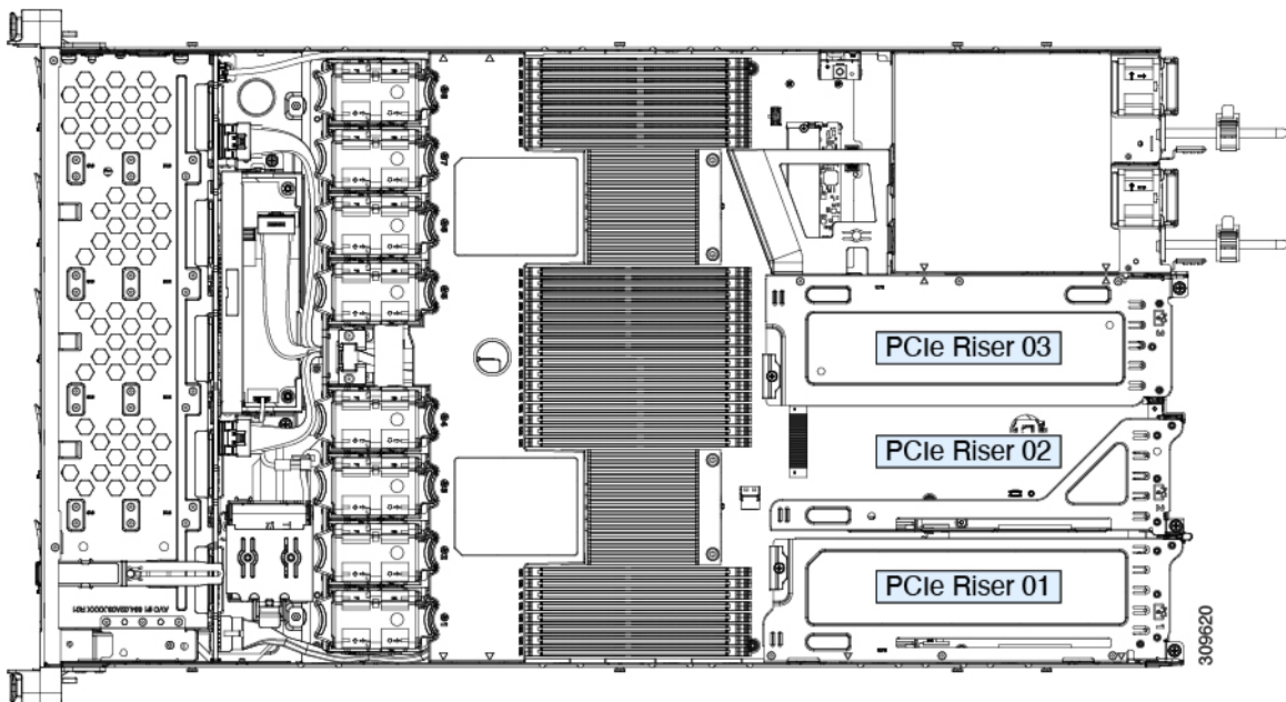
図 29: PCIe ライザーの配置 : 3 ライザー構成
