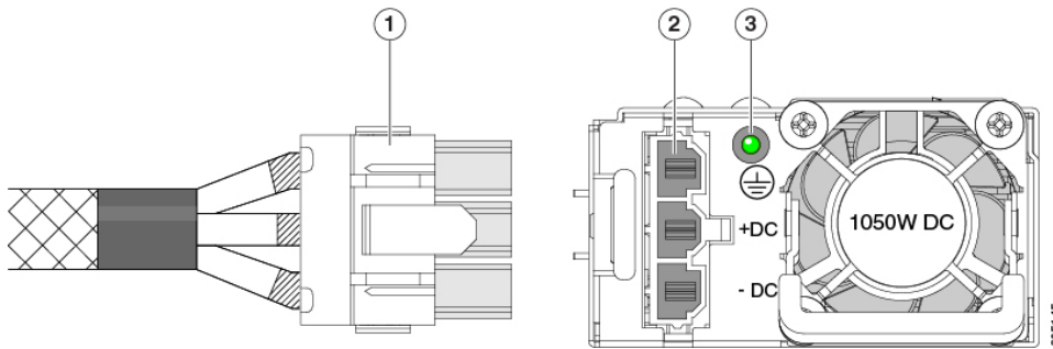
図 27: DC 電源装置の取り付け
