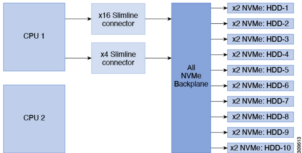
図 45: すべての NVMe バックプレーン
