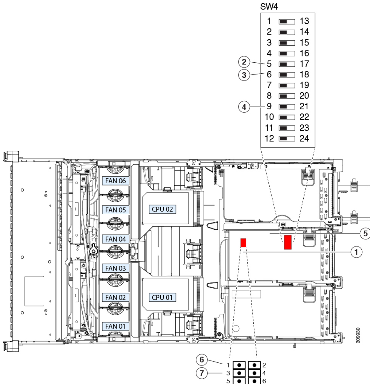
図 41: DIP スイッチおよびサービス ヘッダー ブロック SW4 および CN4 の場所
