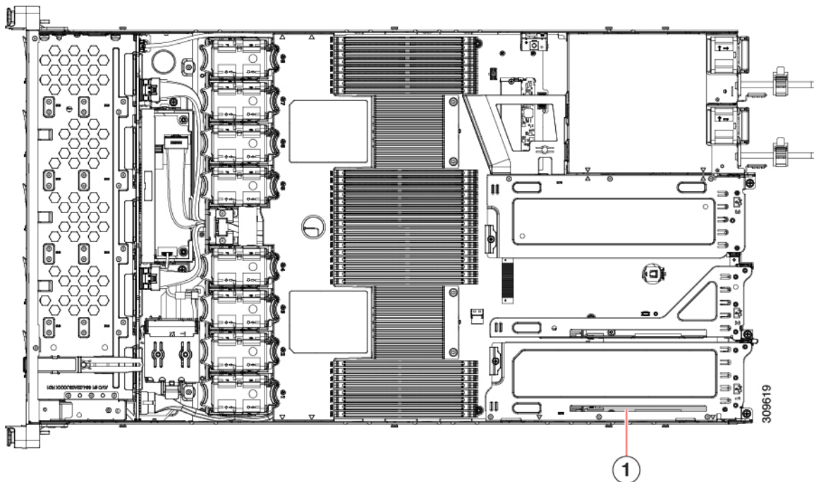
図 35: mLOM カードの位置
