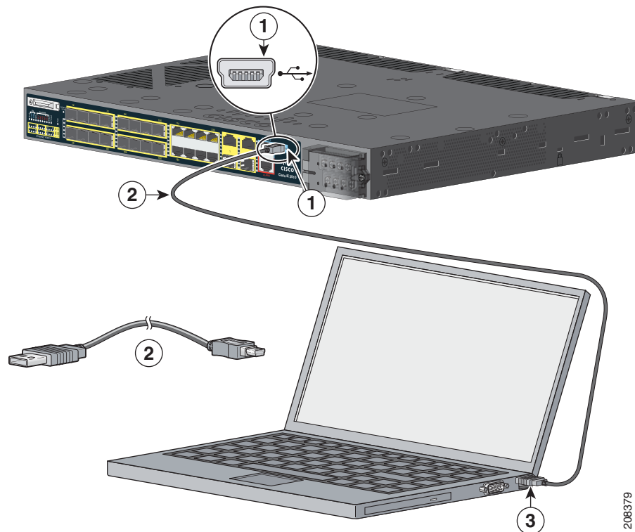
図 42 USB コンソール ケーブルの接続
