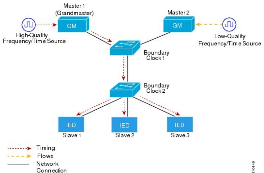
図 1: PTP ネットワーク
