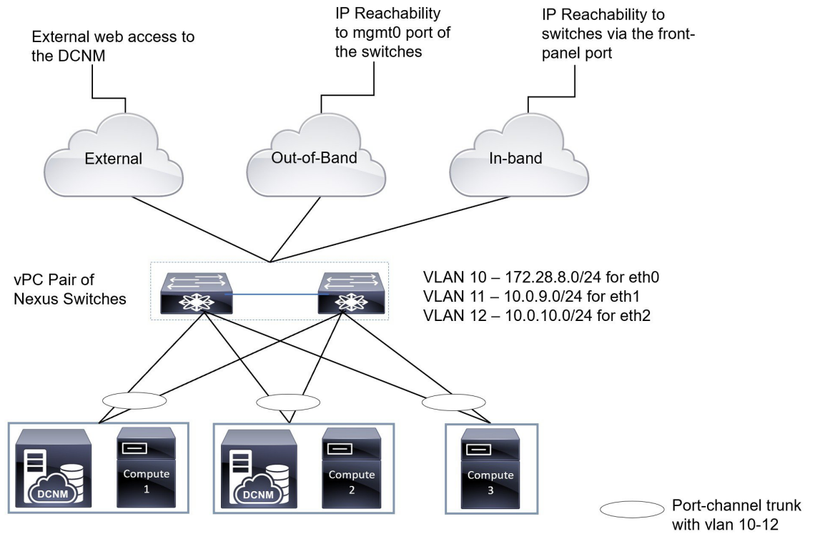
図 19: 3 台のサーバを使用した Cisco DCNM VM の物理接続
