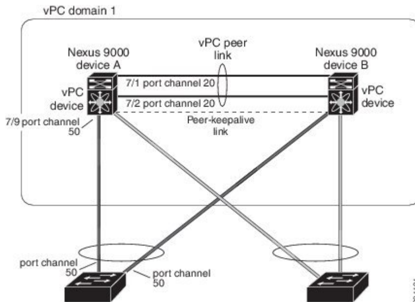
図 18: vPC の設定例
