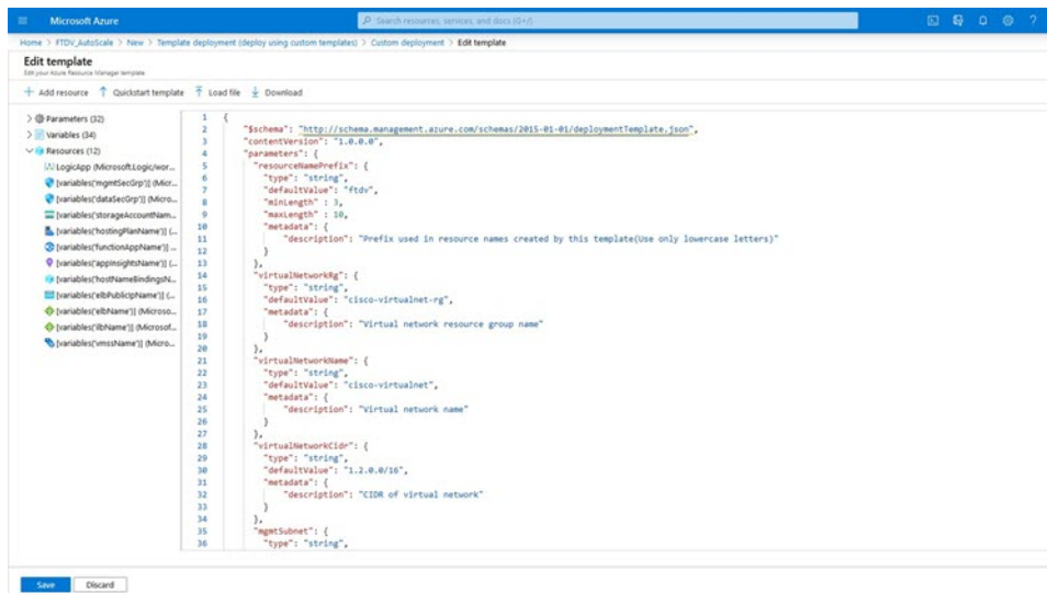
図 16: Edit Template
