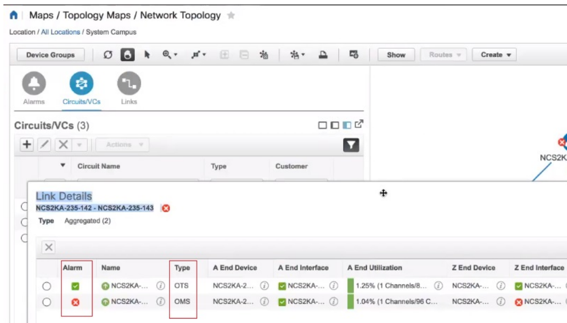
図 6: アラームを使用した [リンクの詳細 (Link Details) ]
