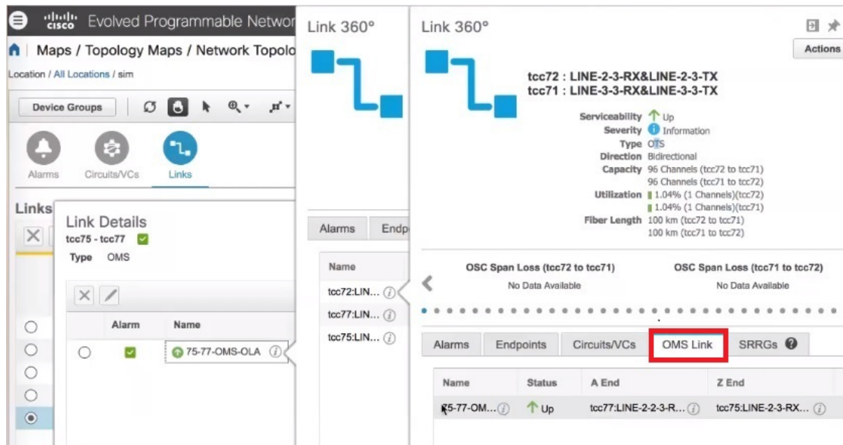
図 5:[リンクの詳細 (Link Details) ]と [リンク 360* (Link 360*) ]ビュー
