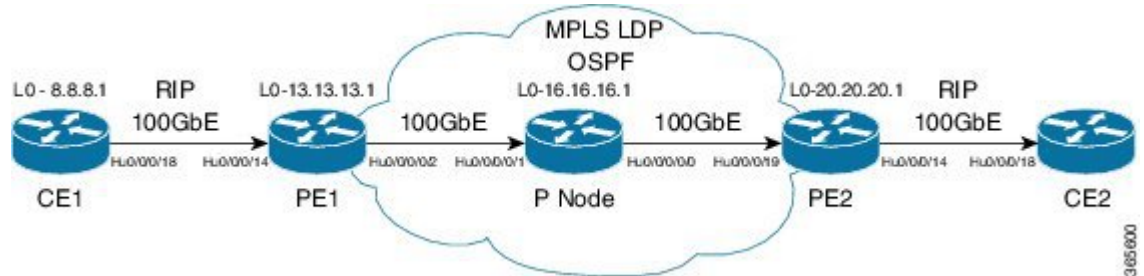
図 4: MPLS LDP を介した L3VPN
