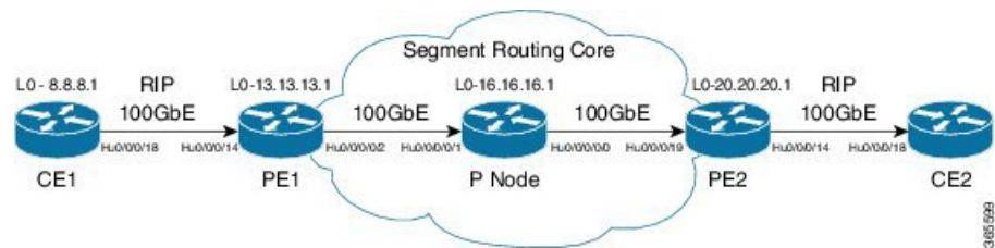
図 10: セグメントルーティングを介した MPLS L3VPN
