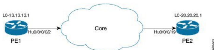
図 6: PE ルータ上での Multiprotocol BGP
