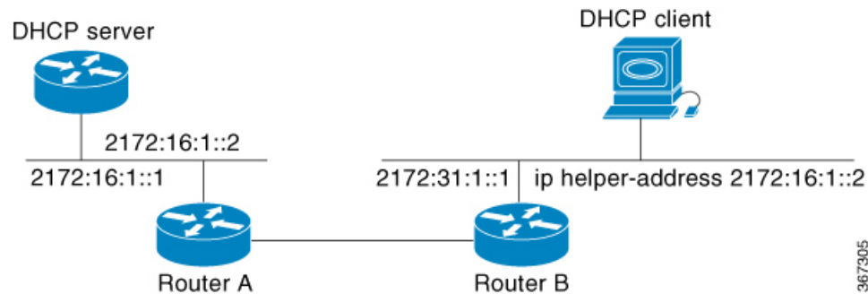
図 11: ヘルパー アドレスを使用した UDP ブロードキャストの DHCPv6 サーバへの転送
