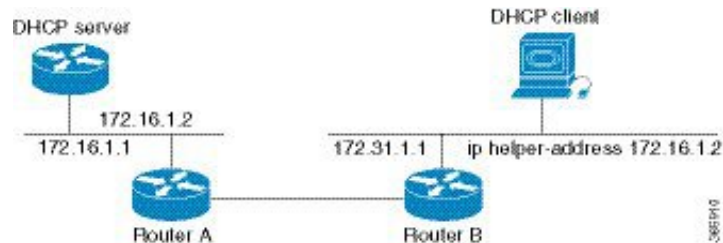
図 10: ヘルパー アドレスを使用した UDP ブロードキャストの DHCP サーバへの転送
