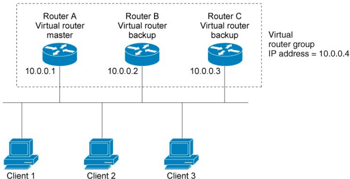
図 12: 基本的な VRRP トポロジ
