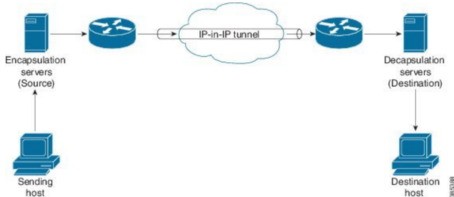
図 11: IP-in-IP トンネルを使用した基本的なカプセル化とカプセル化解除
